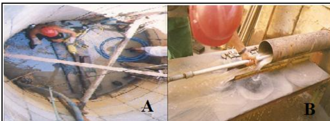
Foto 3 – (A) Inserindo os tubos 6.5/8” horizontalmente na captação; (B) Injeção de água a alta pressão para remoção do material acumulado nos tubos
