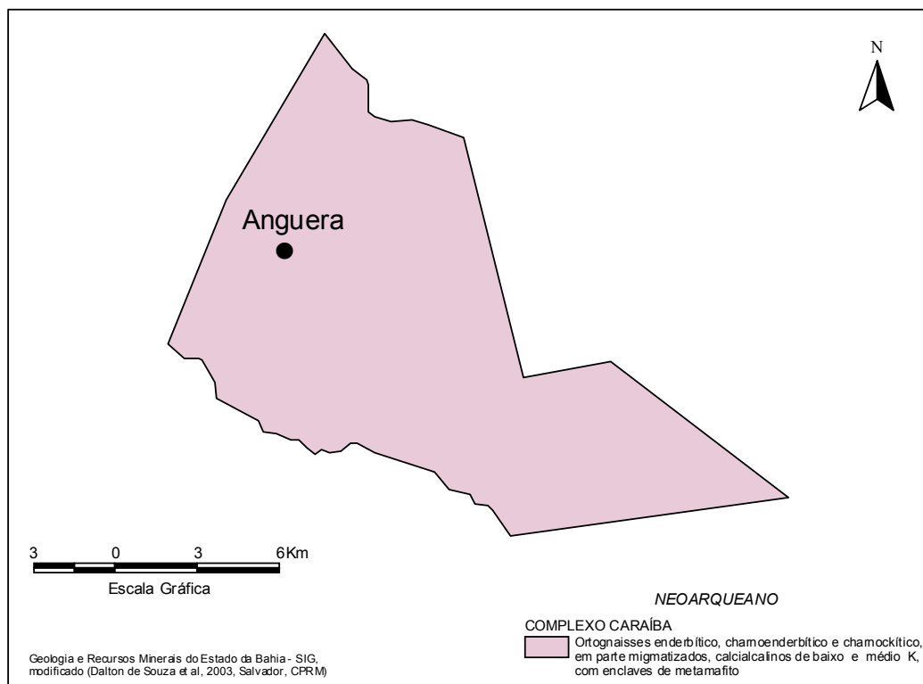
Figura 3 – Esboço geológico.
