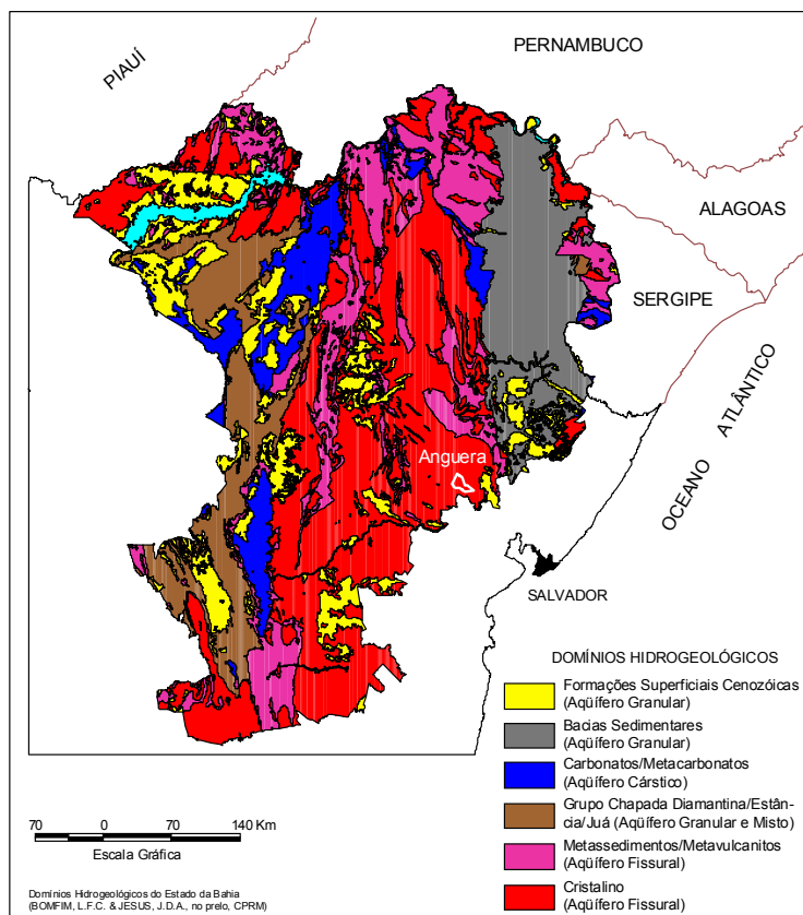
Figura 4 – Domínio hidrogeológico.
