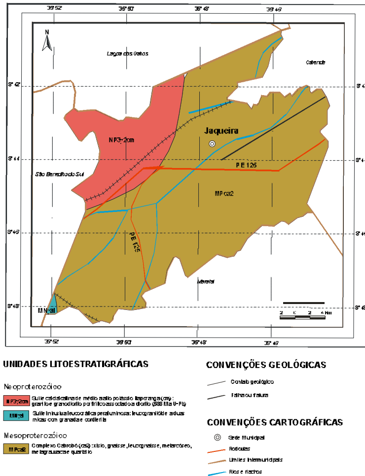
Figura 3 – Mapa Geológico
