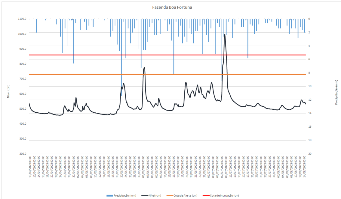
Figura 25 – Nível do rio Mundaú e precipitação na PCD da estação Fazenda Boa Fortuna no município de Rio Largo – AL no período de 10/04/23 à 15/08/23. Fonte: Elaborada pela autora.
