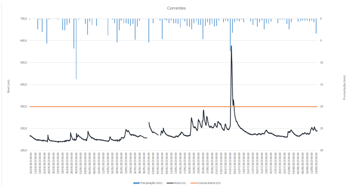
Figura 20 – Nível do rio Mundaú e precipitação na PCD da estação Correntes no município de Correntes – PE no período de 10/04/23 à 15/08/23. Fonte: Elaborada pela autora.
