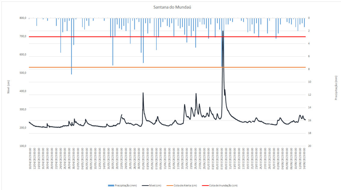
Figura 21 – Nível do rio Mundaú e precipitação na PCD da estação Santana do Mundaú no município de Santana do Mundaú – AL no período de 10/04/23 à 15/08/23. Fonte: Elaborada pela autora.
