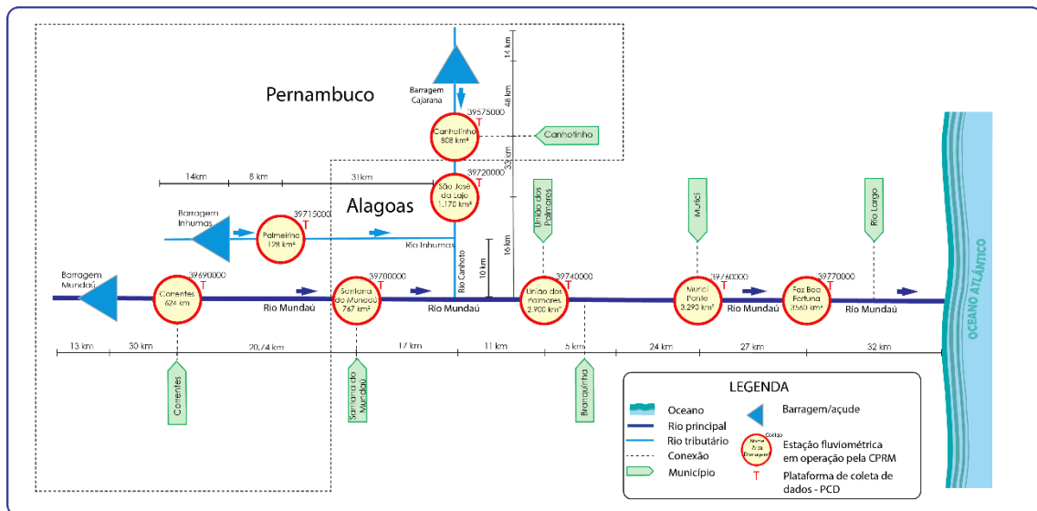
Figura 2 - Diagrama unifilar da bacia do rio Mundaú. Fonte: Elaborada pela autora.
