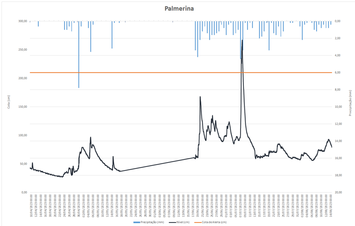
Figura 19 – Nível do rio Inhumas e precipitação na PCD da estação Palmerina no município de Palmerina – PE no período de 10/04/23 à 15/08/23. Fonte: Elaborada pela autora.
