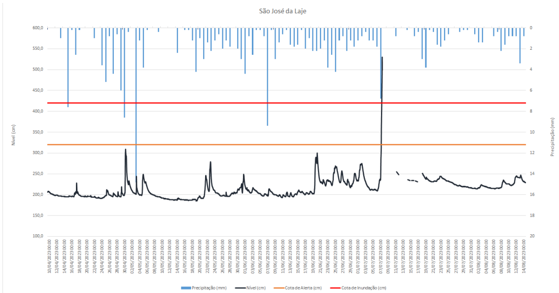
Figura 22 – Nível do rio Canhoto e precipitação na PCD da estação São José da Laje no município de São José da Laje – AL no período de 10/04/23 à 15/08/23. Fonte: Elaborada pela autora.
