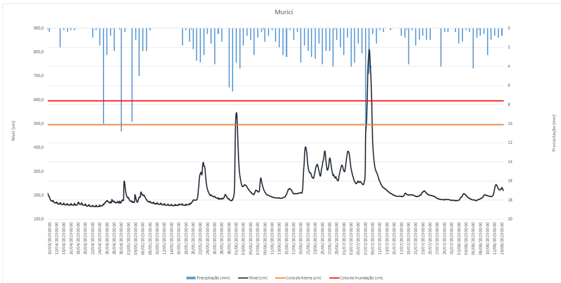
Figura 24 – Nível do rio Mundaú e precipitação na PCD da estação de Murici-Ponte no município de Murici – AL no período de 10/04/23 à 15/08/23. Fonte: Elaborada pela autora.
