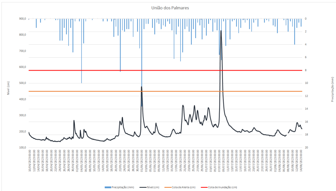
Figura 23 - Nível do rio Mundaú e precipitação na PCD da estação de União dos Palmares no município de União dos Palmares – AL no período de 10/04/23 à 15/08/23. Fonte: Elaborada pela autora.
