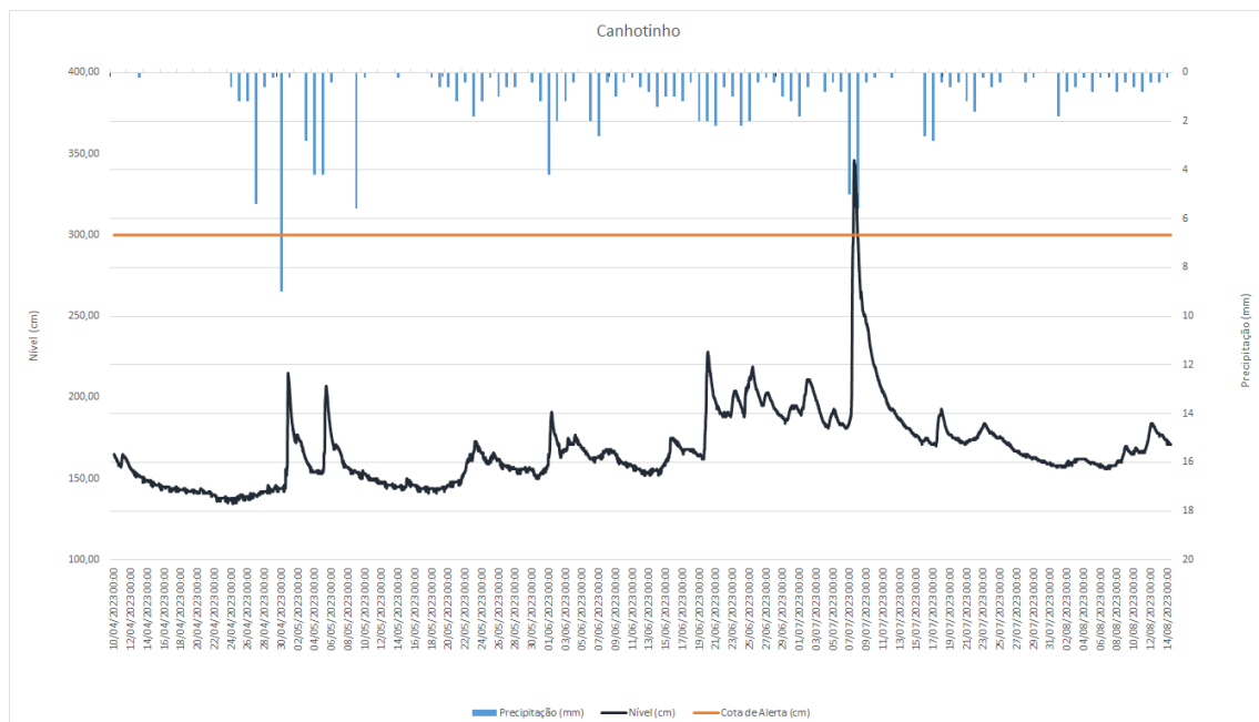
Figura 18 – Nível do rio Canhoto e precipitação na PCD da estação Canhotinho no município de Canhotinho – PE no período de 10/04/23 à 15/08/23. Fonte: Elaborada pela autora.
