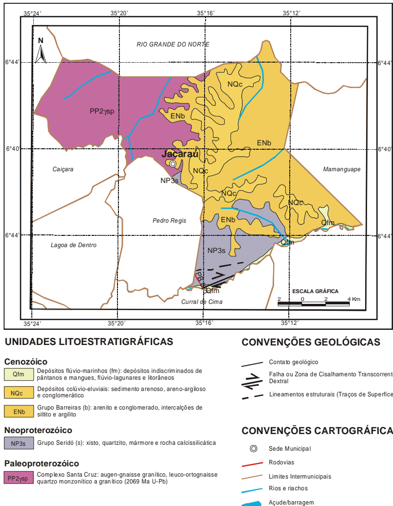
Figura 3 – Mapa Geológico
