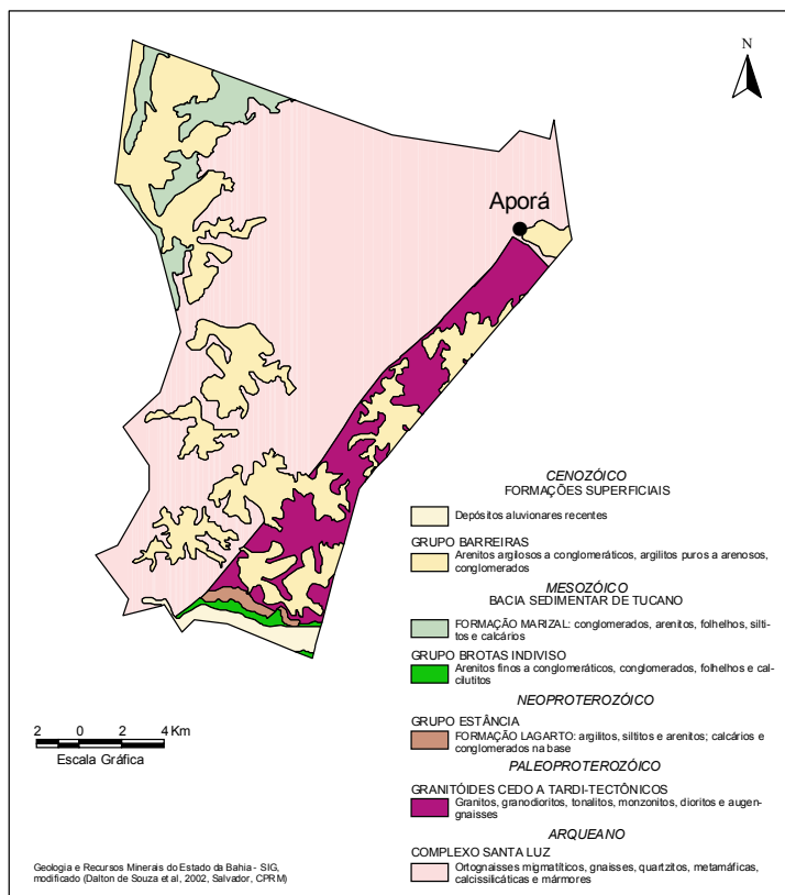
Figura 3 – Esboço geológico.
