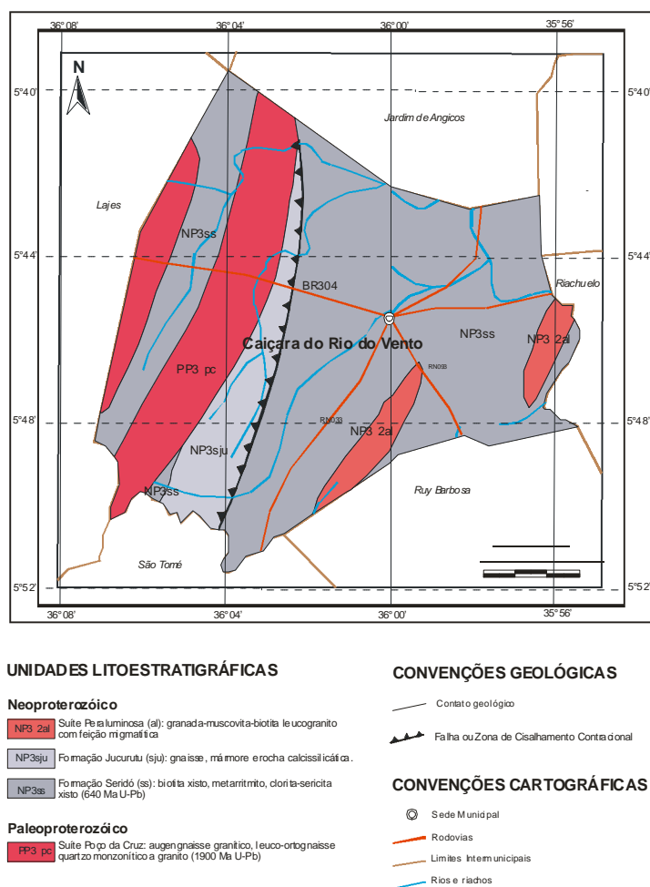
Figura 3 - Mapa Geológico
