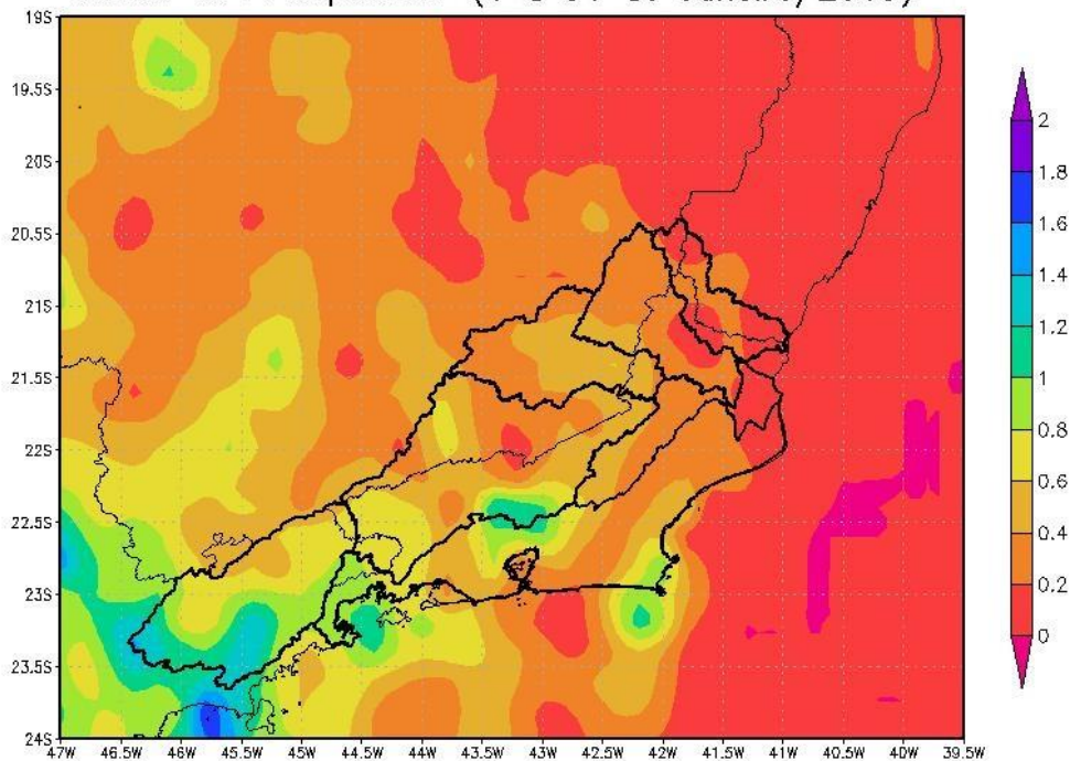
Razao da Precipitacao (1 a 31 de Janeiro/2019)
