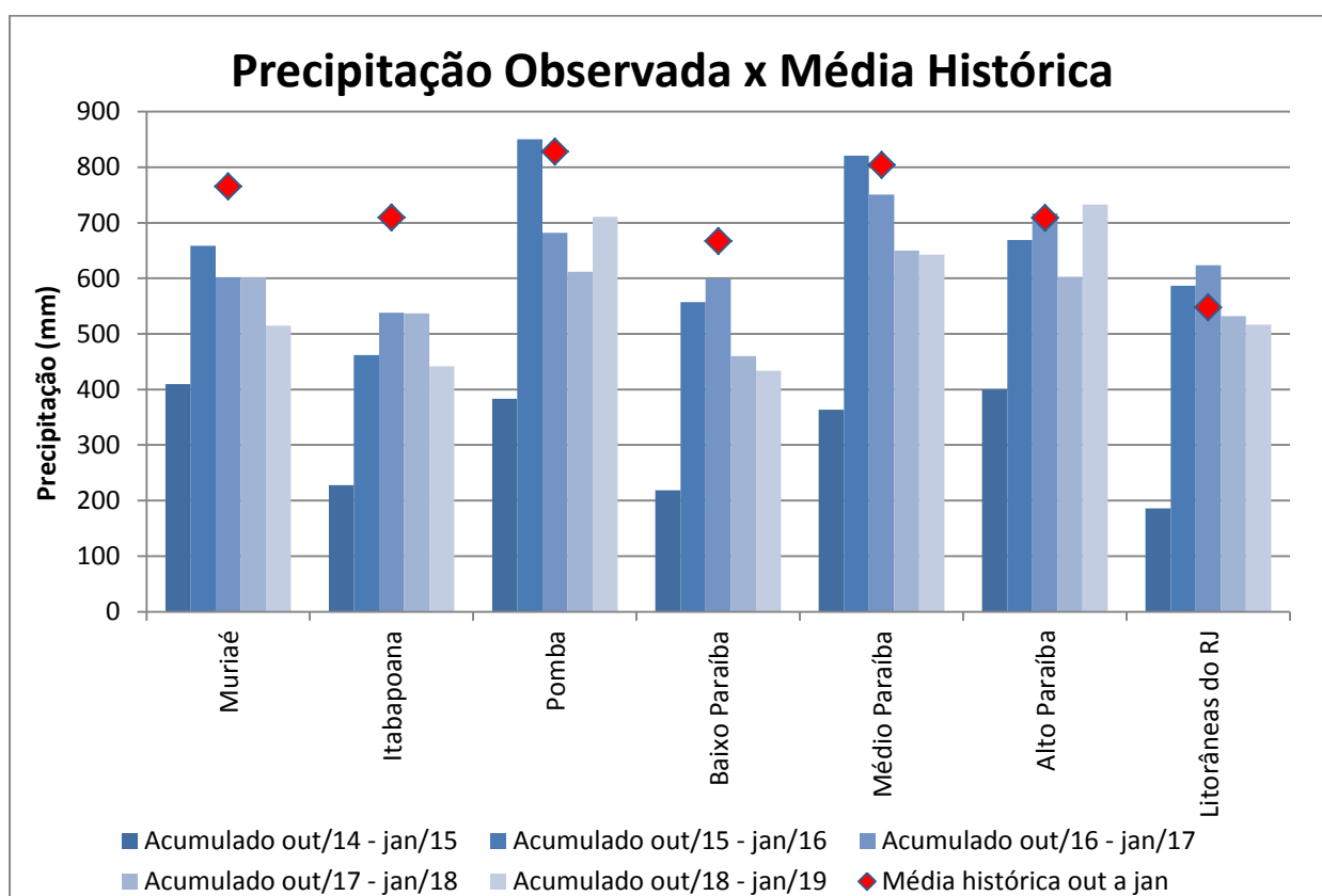
Figura 5 - Comparação entre a precipitação média histórica de outubro a janeiro, e a precipitação acumulada de outubro a janeiro de 2015, 2016, 2017, 2018 e 2019 nas bacias da área de atuação da SUREG/SP.
