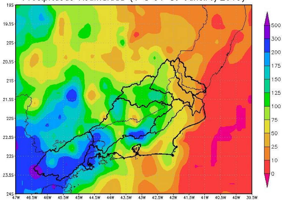
Precipitacao Acumulada (1 a 31 de Janeiro/2019)
