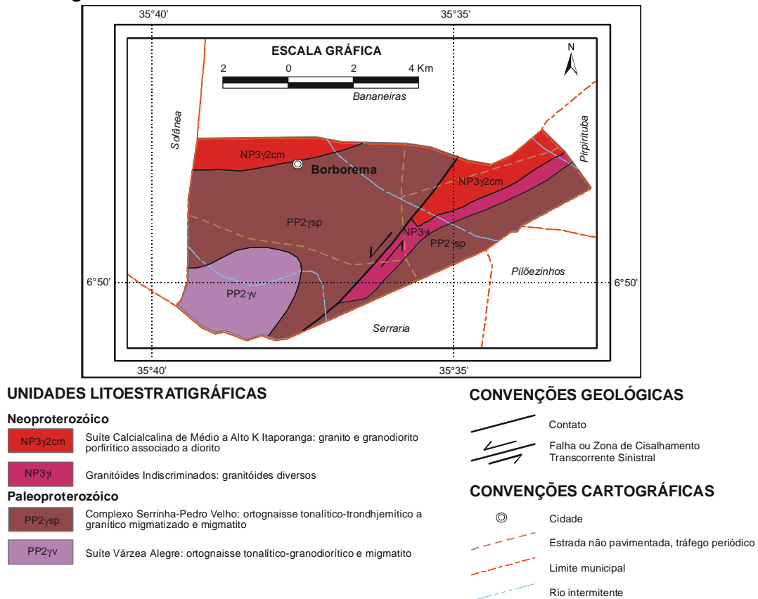
Figura 3 – Mapa Geológico
