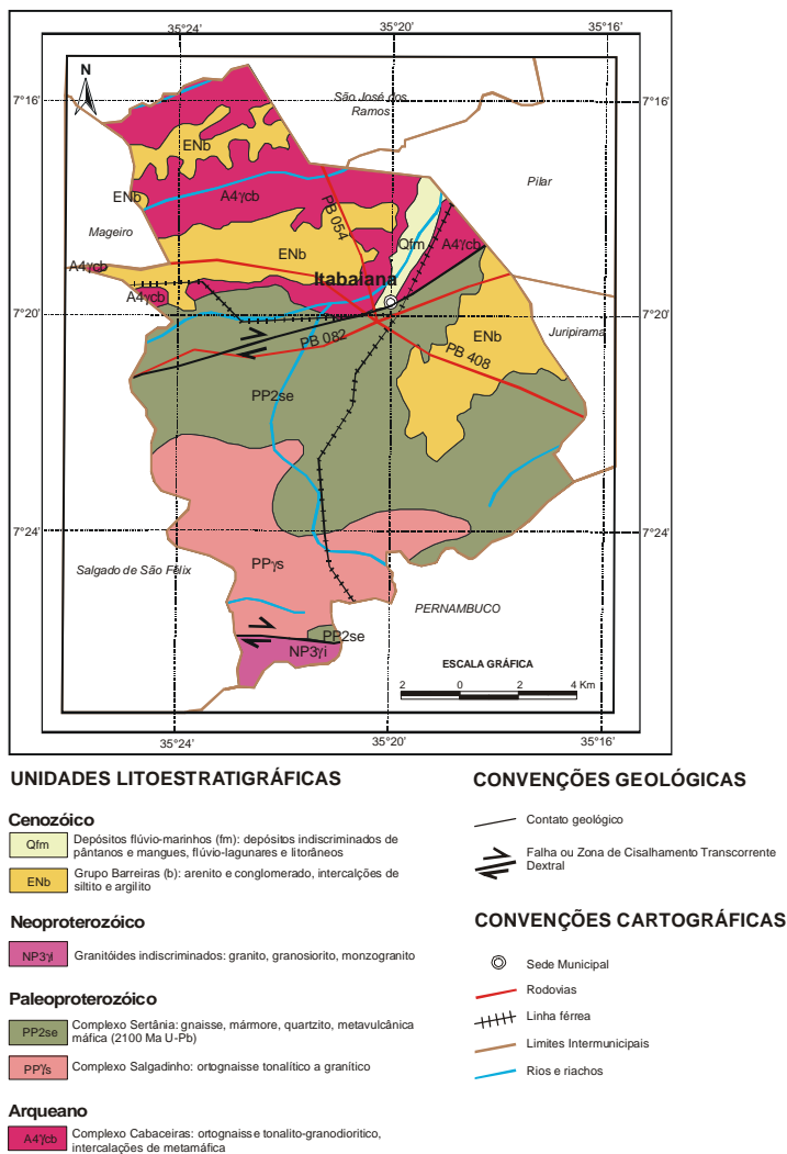
Figura 3 – Mapa Geológico
