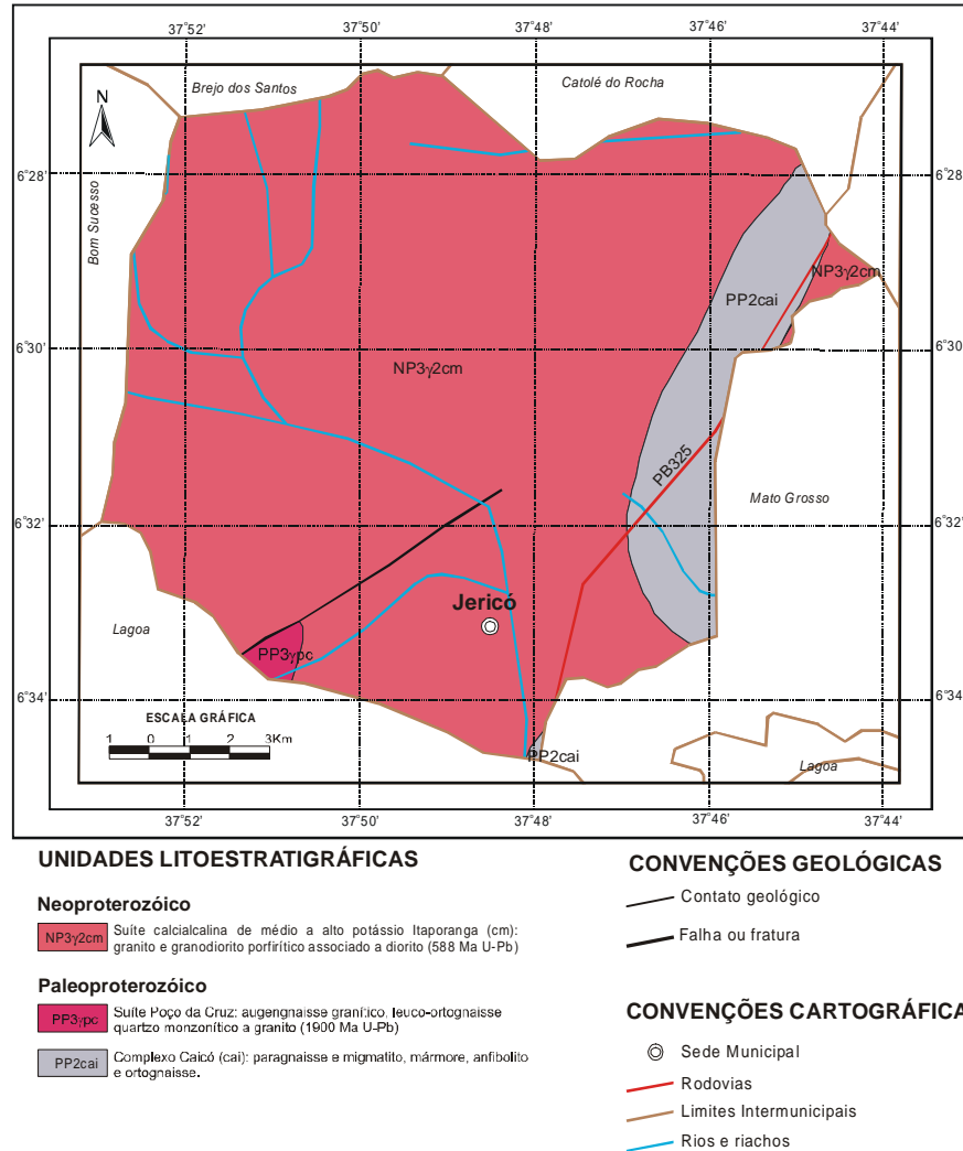
Figura 3 – Mapa Geológico
