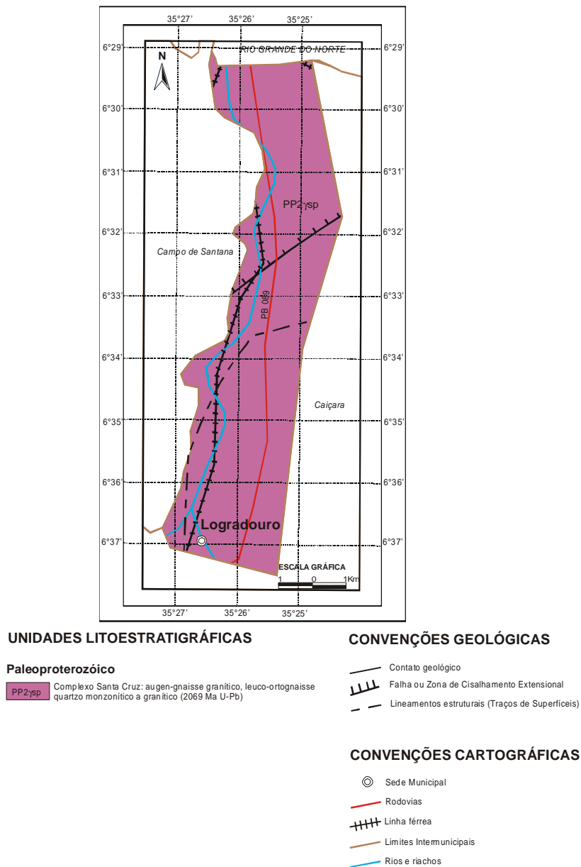
Figura 3 – Mapa Geológico
