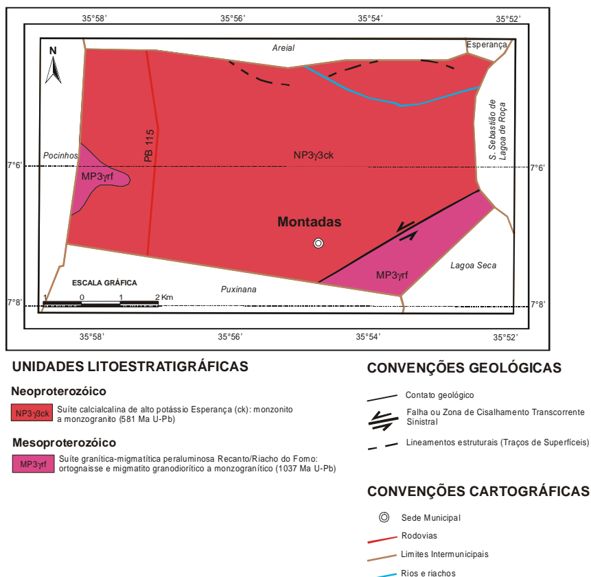
Figura 3 – Mapa Geológico
