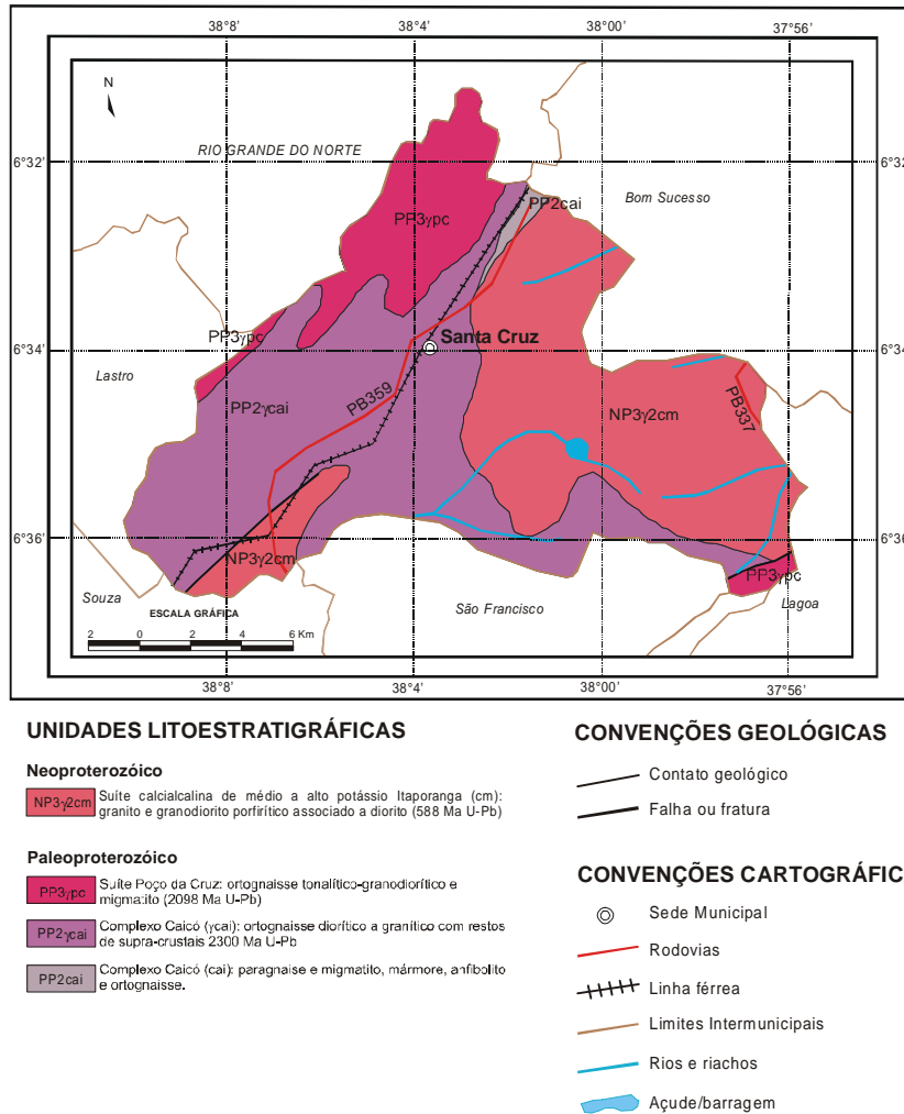
Figura 3 – Mapa Geológico
