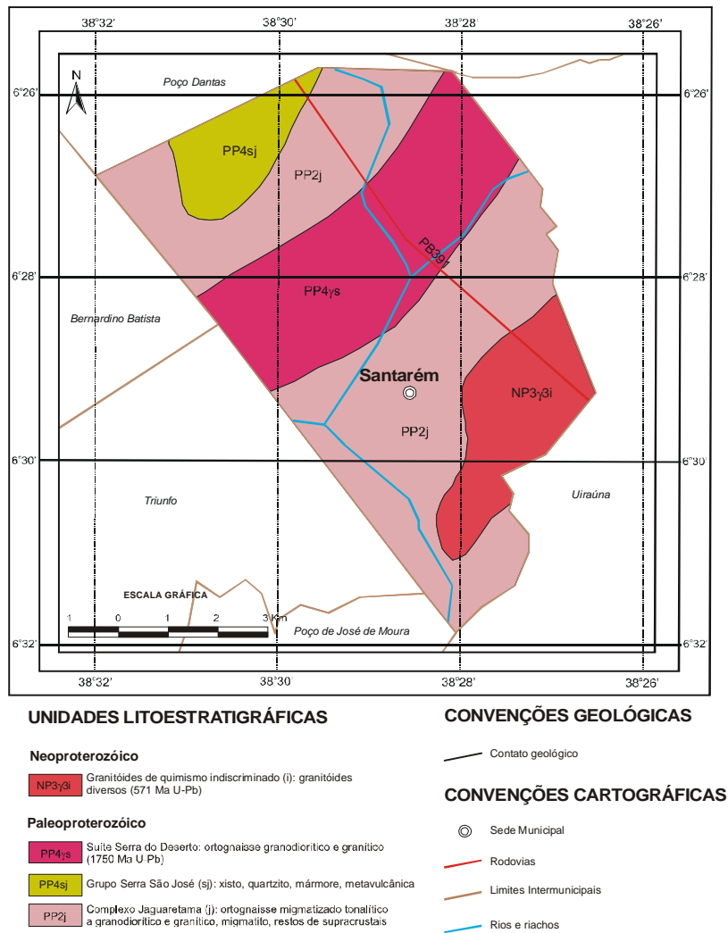
Figura 3 – Mapa Geológico
