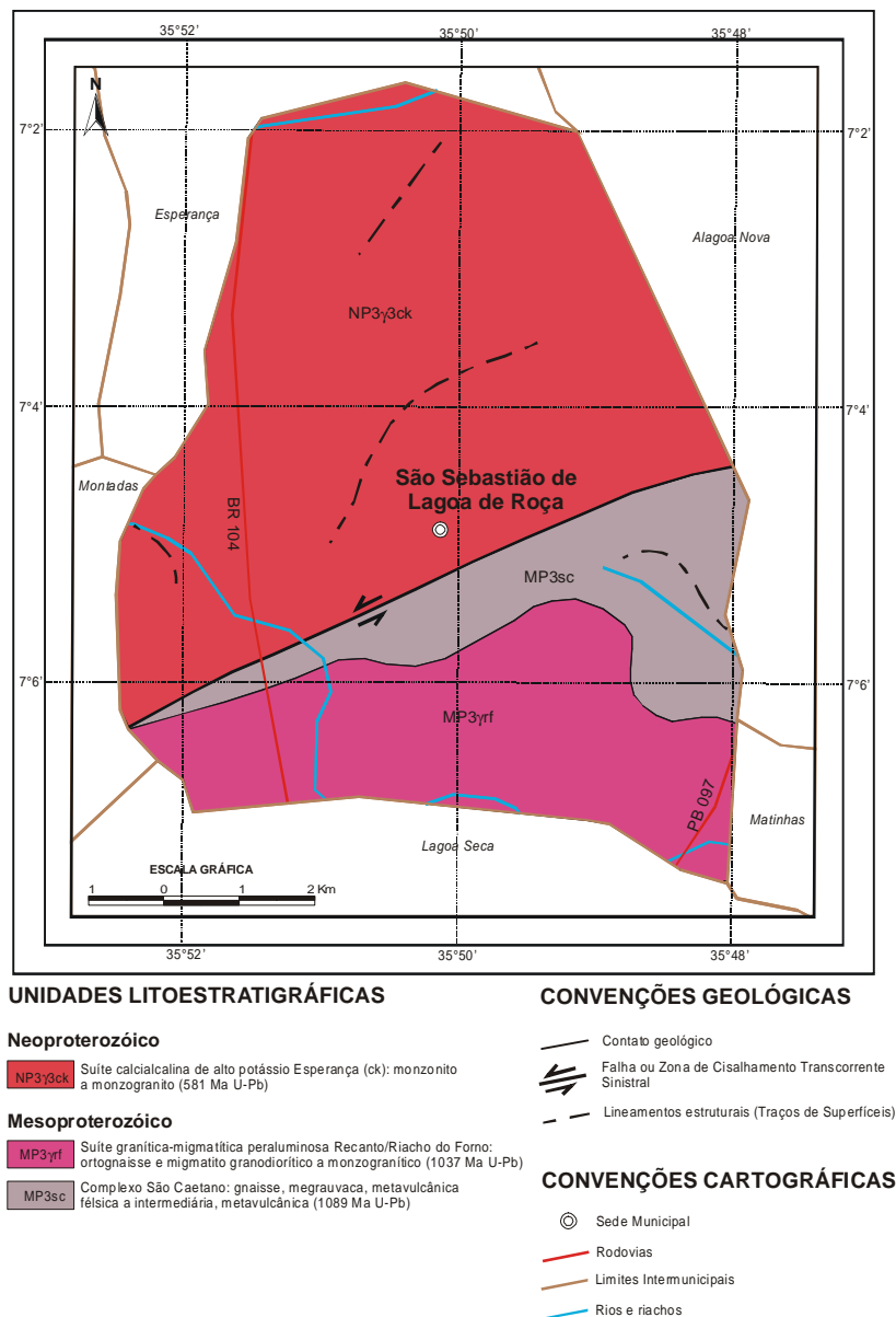
Figura 3 – Mapa Geológico
