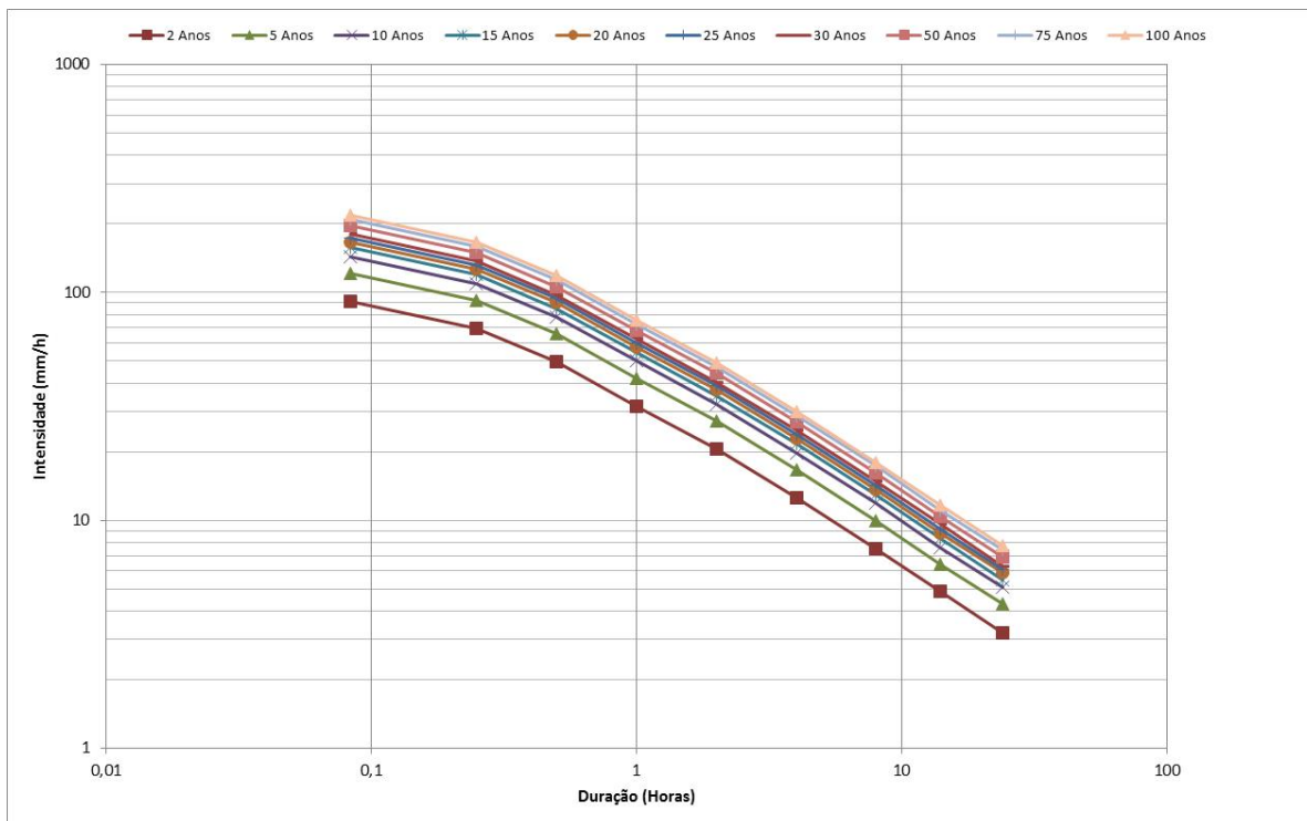
Figura 02 – Curvas intensidade-duração-frequência
