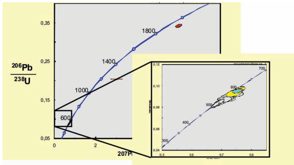
Figura 5.27 - Diagrama concórdia para a amostra TJ-46 (zircões herdados em vermelho). No diagrama ampliado apresenta-se a idade concórdia de 592 \pm 7 Ma. Apenas as análises representadas pelas elipses preenchidas (amarelo) foram utilizadas no cálculo da idade concórdia (elipse preenchida de azul)
