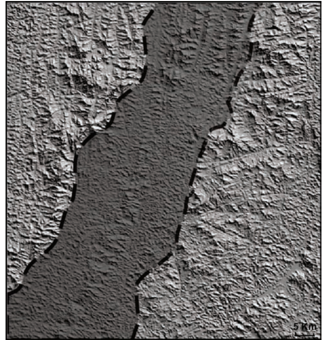
Figura 5.11 - Imagem de relevo sombreado da Folha Carangola, em destaque o domínio estrutural da Zona de Cisalhamento de Manhauçu
