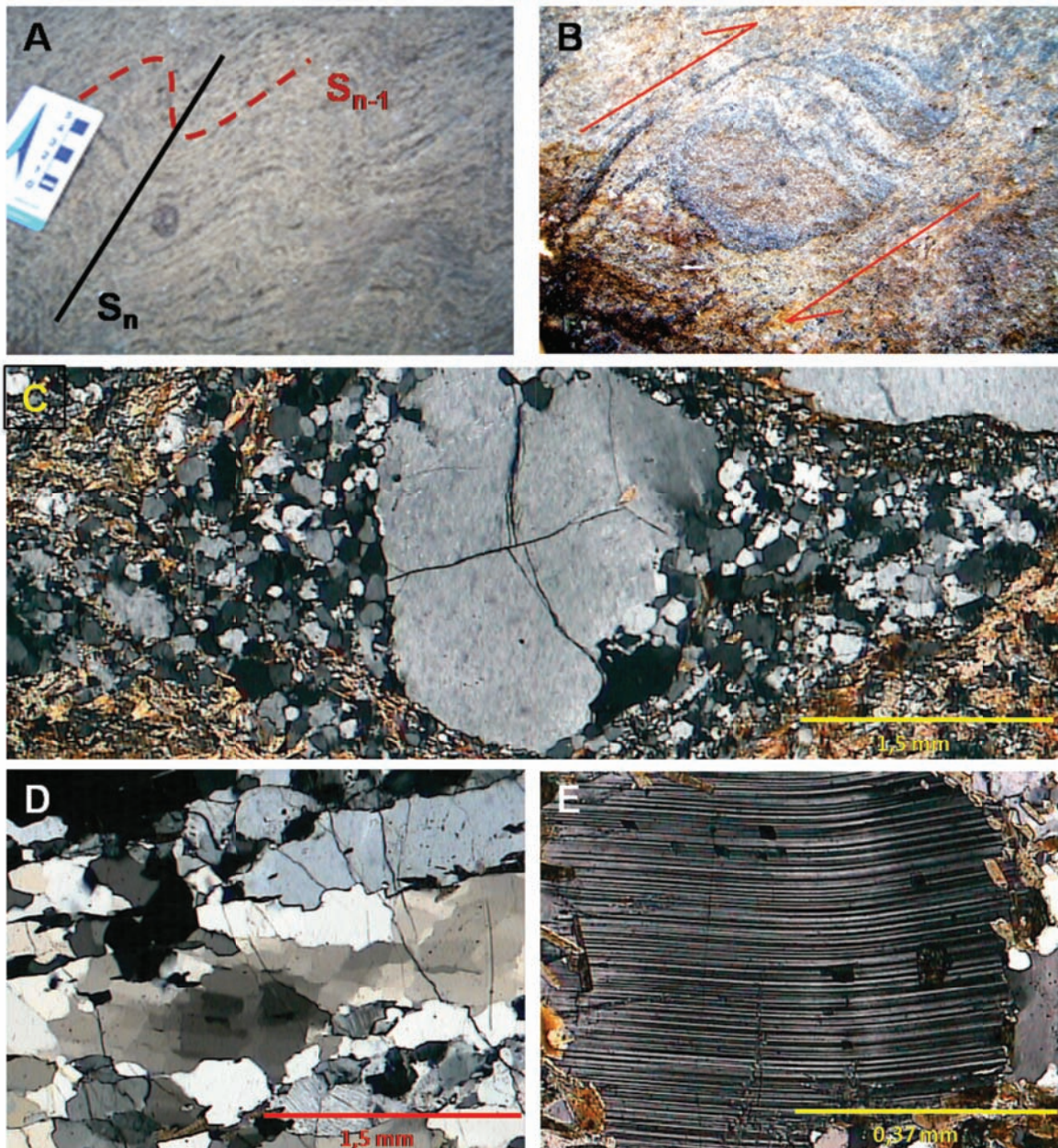
Figura 5.14 - A) Preservação de foliação mais antiga ( S_{n-1} ) no ortognaisse do Complexo Juiz de Fora (Ponto 1479, 7714865N/806449E). Feições de deformação e milonitização relacionadas ao cisalhamento durante a fase D2: B) Indicador cinemático em paragneisse do Grupo Andrelândia (Ponto 998, 7703544N/809687E); C) Fotomicrografia de porfiroclasto de feldspato potássico pertítico exibindo sombra de pressão e cauda de recristalização em paragneisse milonítico do Grupo Andrelândia; nicóis cruzados (Ponto 1570, 7711961N/791543E); D) Fotomicrografia de quartzo fitado, subgranulado e com extinção ondulante em granito porfirítico milonitizado da Suíte Pangarito, nicóis cruzados (Ponto 1450, 7712870N/794052E); E) Fotomicrografia de cristal de plagioclásio com macla recurvada em paragneisse do Grupo Andrelândia; nicóis cruzados (Ponto 1571, 7715763N/794437E)
