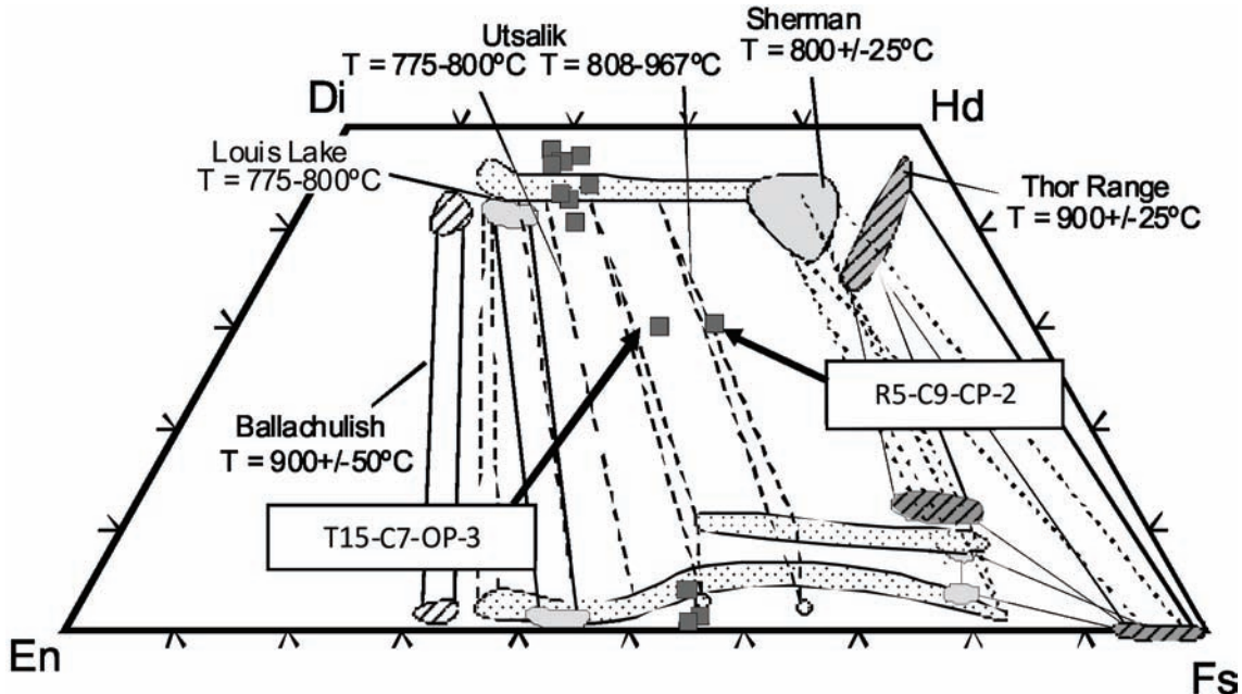
Figura 5.10 - Diagrama composicional para análise de química mineral em cristais de piroxênio de amostras da Suíte Leopoldina (quadrados) e algumas suítes charnockíticas do mundo (Frost & Frost 2008)
