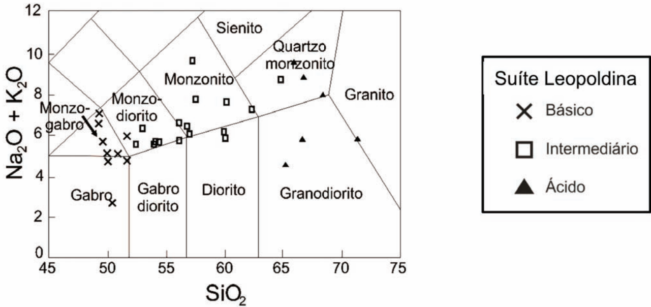
Figura 5.15 - Classificação das amostras da Suíte Leopoldina no diagrama TAS de Wilson (1989) e Xianhua et al. (2000), discriminadas quanto ao conteúdo em sílica (ácidas com teor de SiO_2 > 65\% ; intermediárias 52\% < SiO_2 < 65\% e básicas 45\% < SiO_2 < 52\% )
