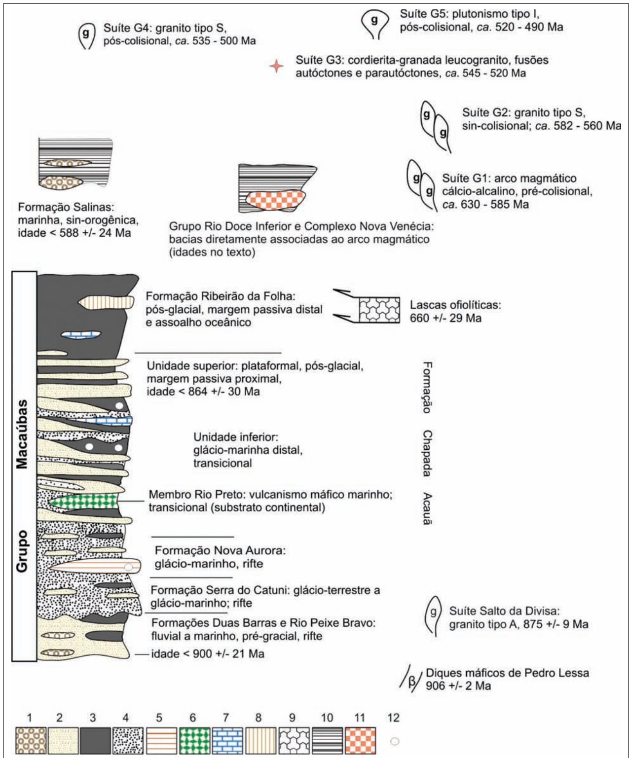
Figura 4.2 - Coluna estratigráfica esquemática do Orógeno Araçuaí. 1, conglomerados; 2, arenitos; 3, pelitos; 4, diamictitos; 5, formação ferrífera diamicítica; 6, basalto transicional; 7, calcário dolomítico; 8, sedimentos exalativos (chert sulfetado, sulfeto maciço, formações ferríferas e outros); 9, rochas máficas (com veios de plagiogranito) e ultramáficas oceânicas; 10, wackes e pelitos; 11, rochas piroclásticas e vulcanoclásticas dacíticas; 12, seixos e blocos pingados (Pedrosa-Soares et al. 2007)
