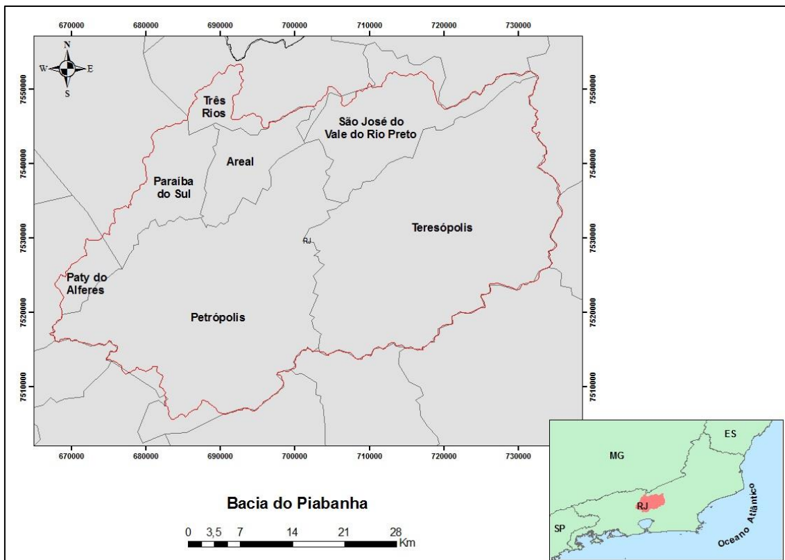
Figura 1.1 - Bacia hidrográfica do rio Piabanha
