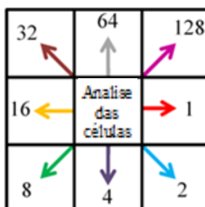
Figura 8.8 - Oito possíveis direções de fluxo no cálculo do aspecto
