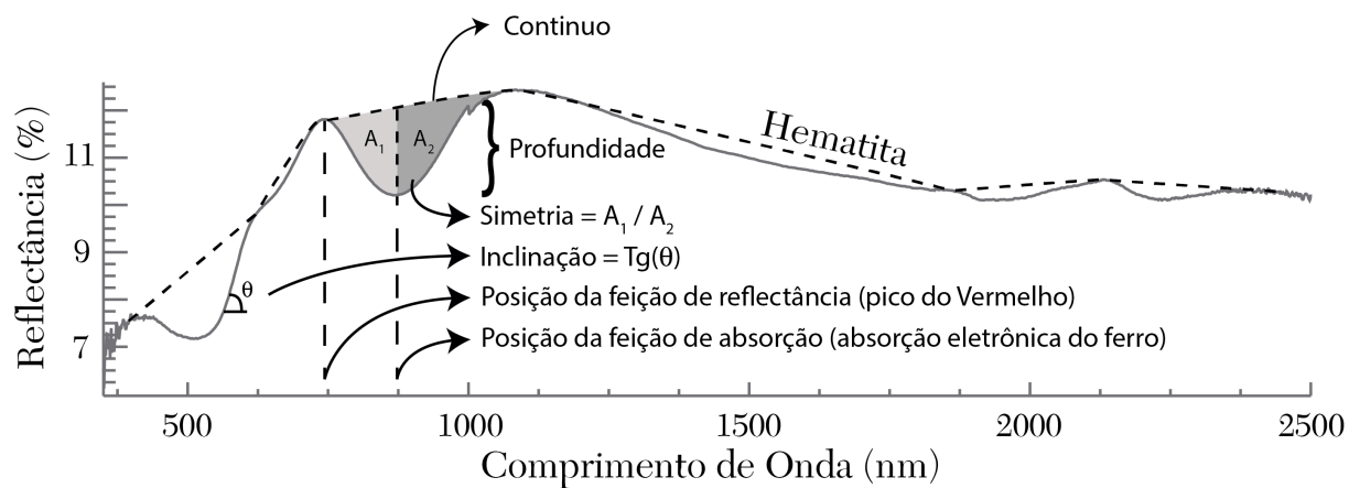
Figura 2.5 Parâmetros espectrais obtidos dos espectros médios de cada método de amostragem.
