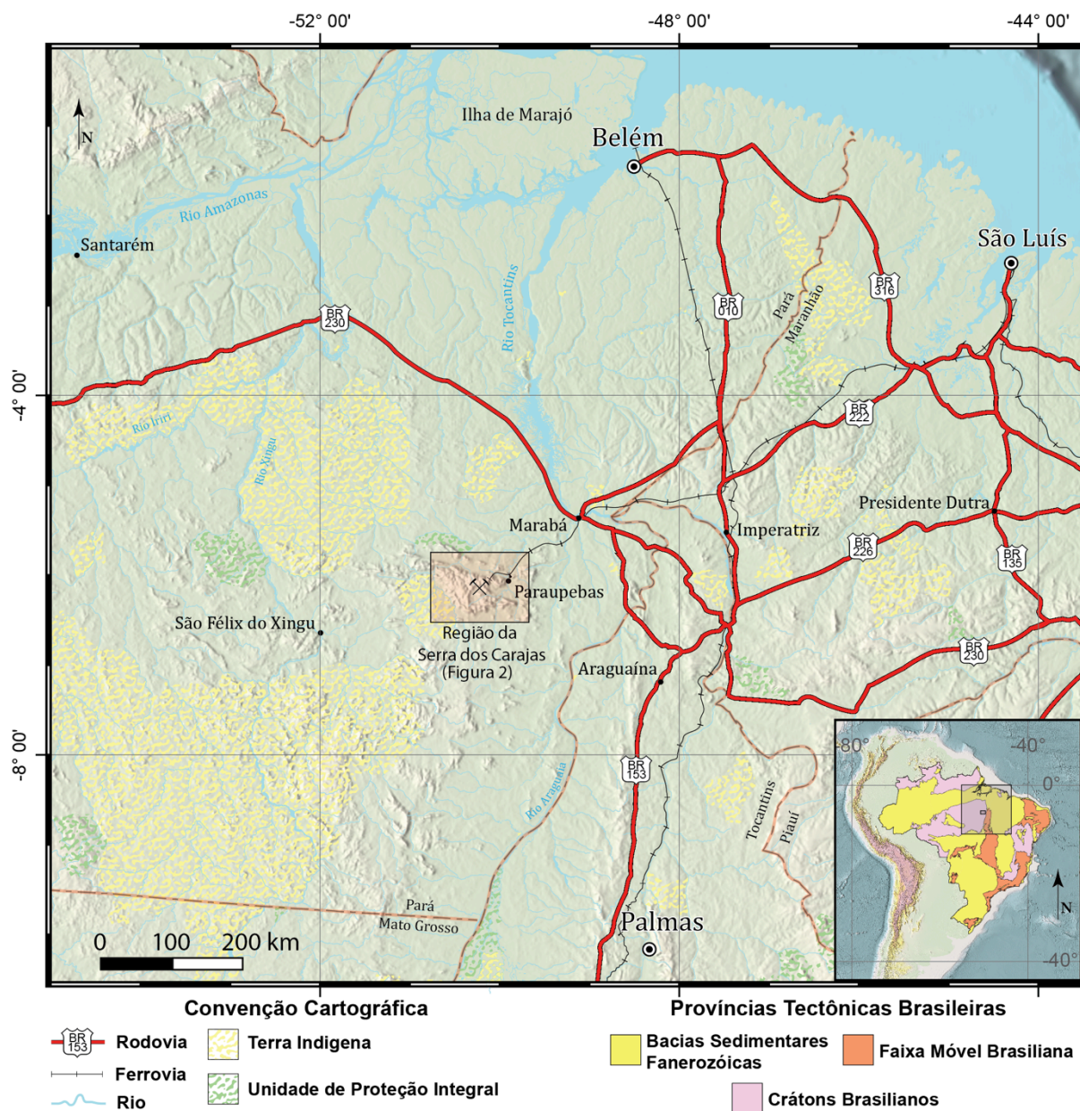
Figura 1.1 Mapa de localização da região da Serra dos Carajás, mostrando as principais vias de acesso, unidades de proteção integral e terras indígenas. No canto inferior direito, apresenta-se a localização da área de estudo em relação às Províncias Tectônicas Brasileiras definidas por Almeida et al. (1977).
