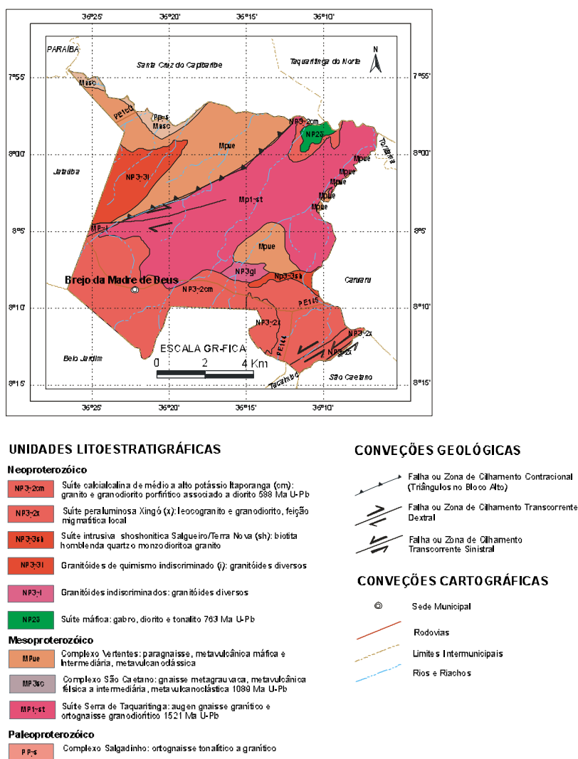
Figura 3- Mapa Geológico
