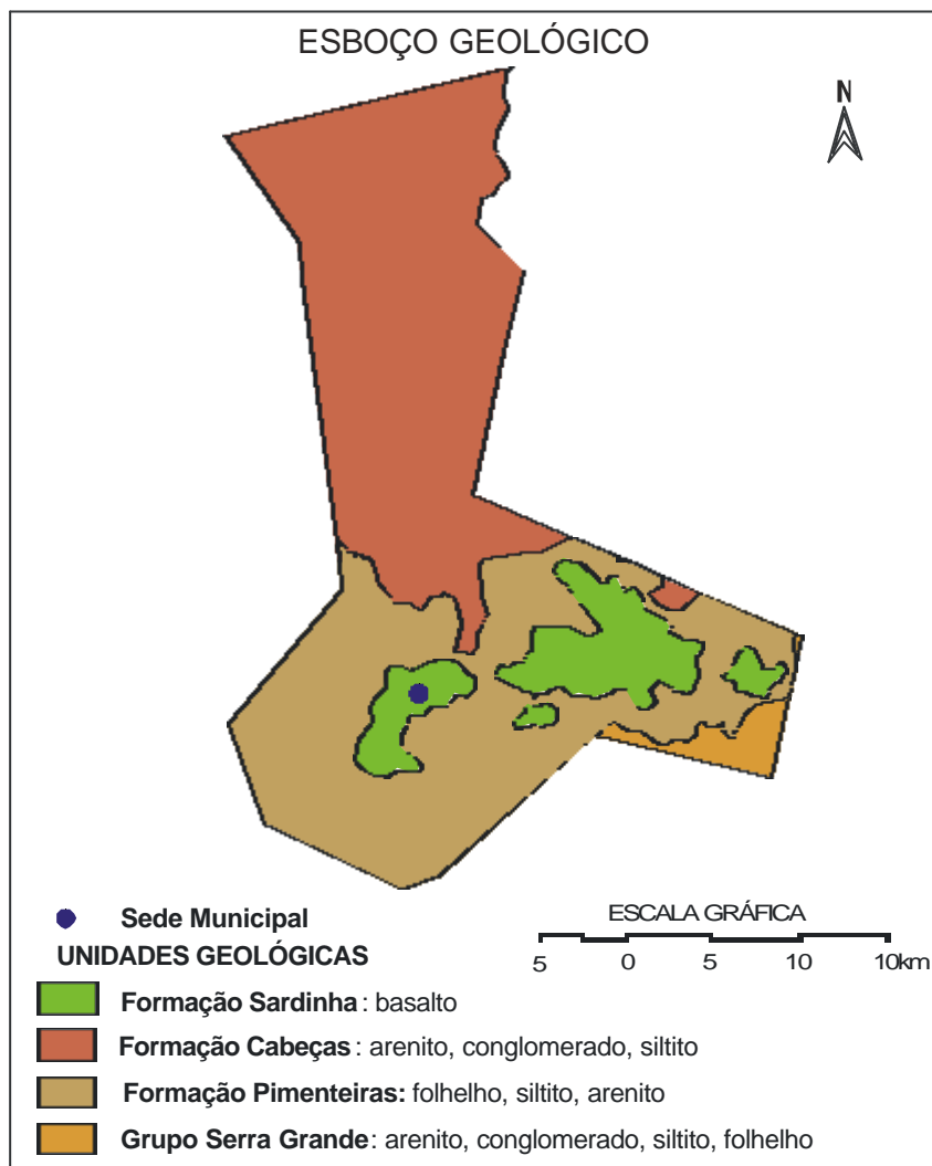
Figura 3 - Esboço geológico do município.
