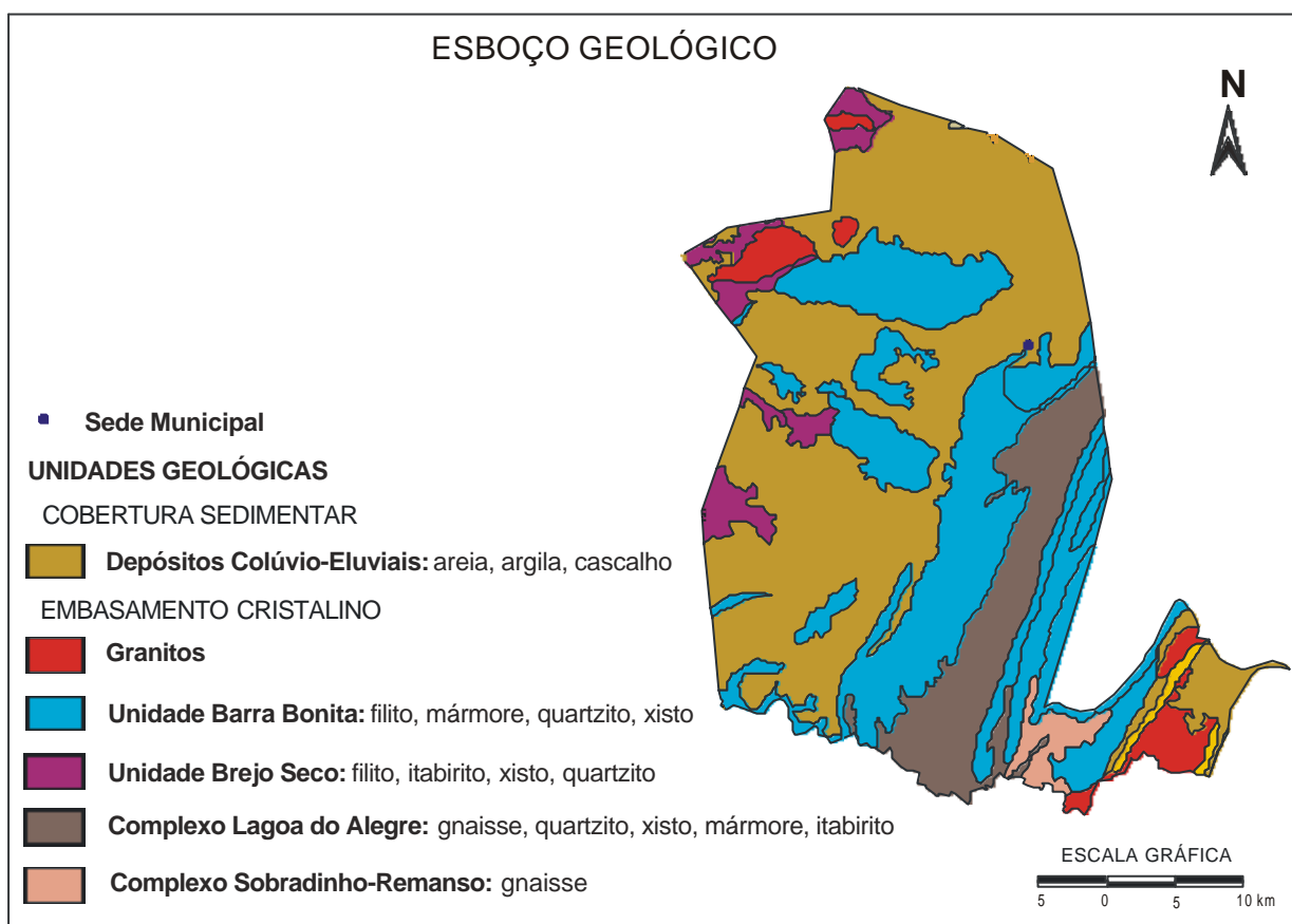
Figura 3 – Esboço geológico do município.
