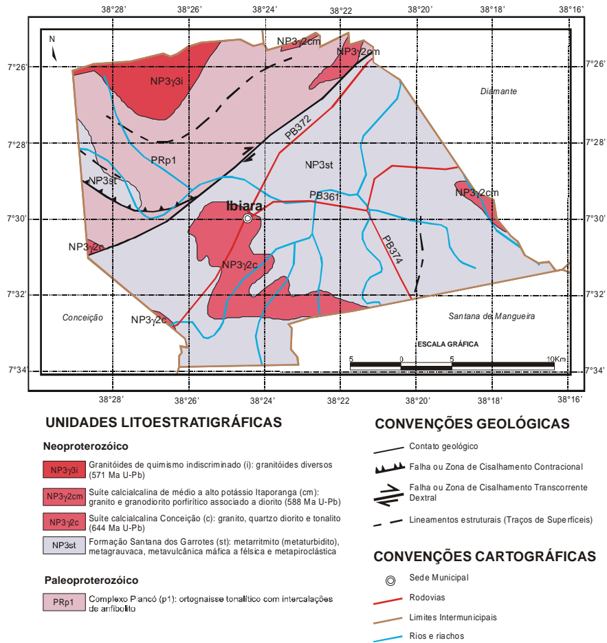
Figura 3 – Mapa Geológico
