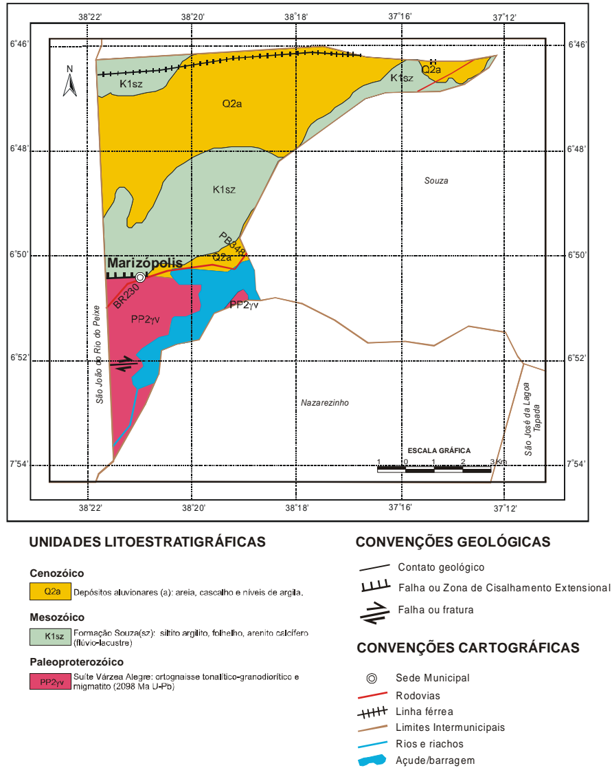
Figura 3 – Mapa Geológico
