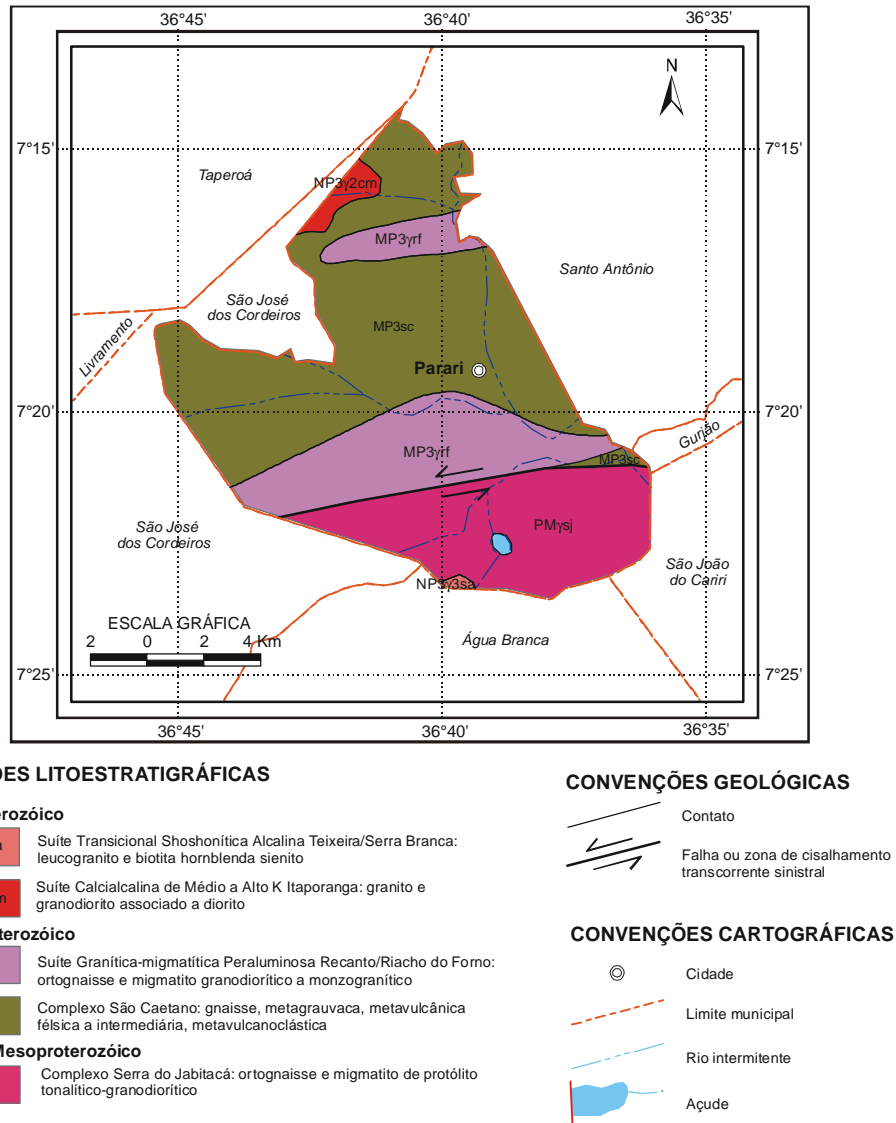
Figura 3 – Mapa Geológico
