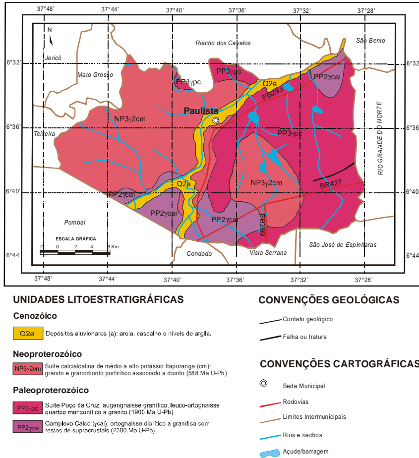
Figura 3 – Mapa Geológico
