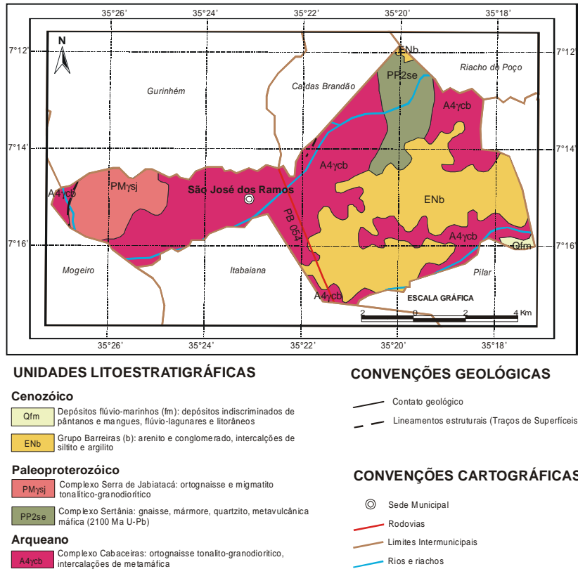
Figura 3 – Mapa Geológico
