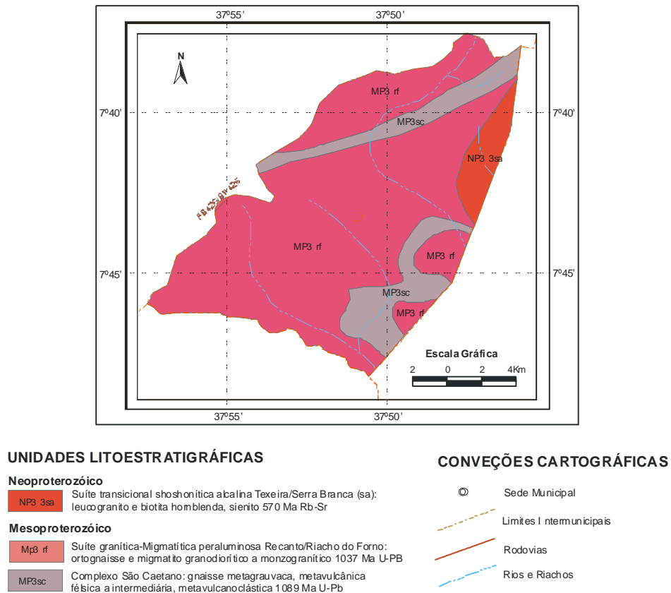
Figura 3- Mapa Geológico
