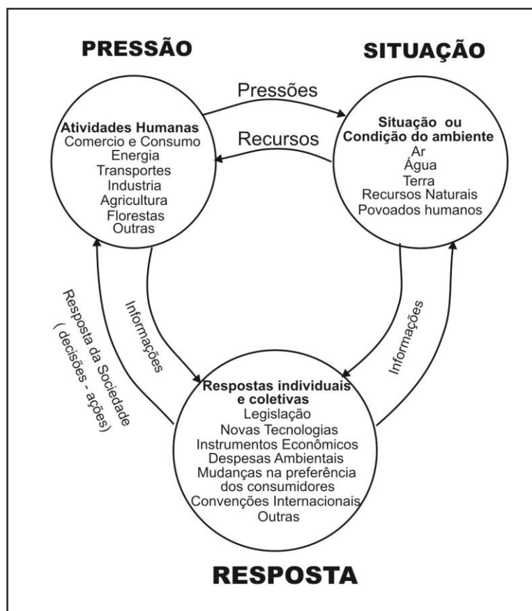
Figura 2.8 Esquema pressão-estado-resposta
