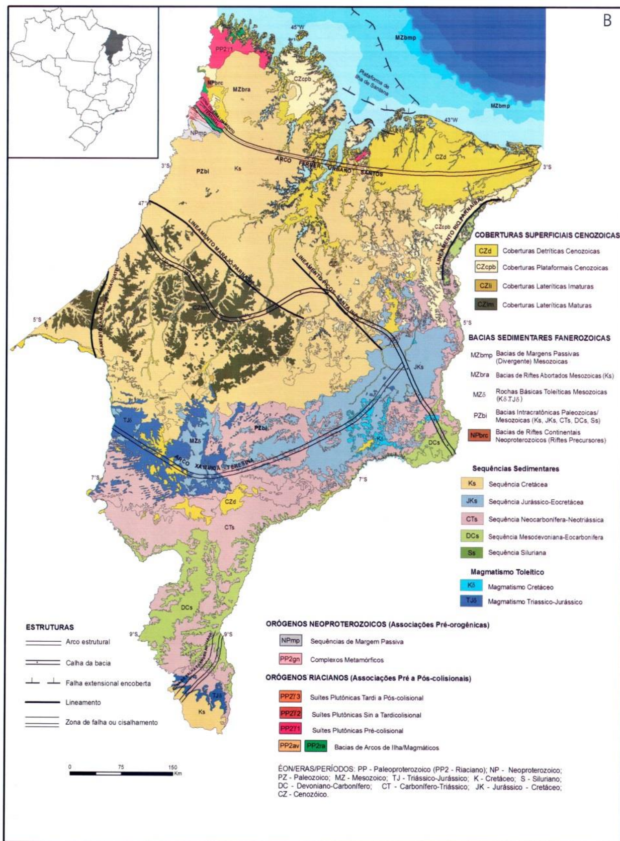
Figura 4.5 Mapa tectônico do Maranhão.
