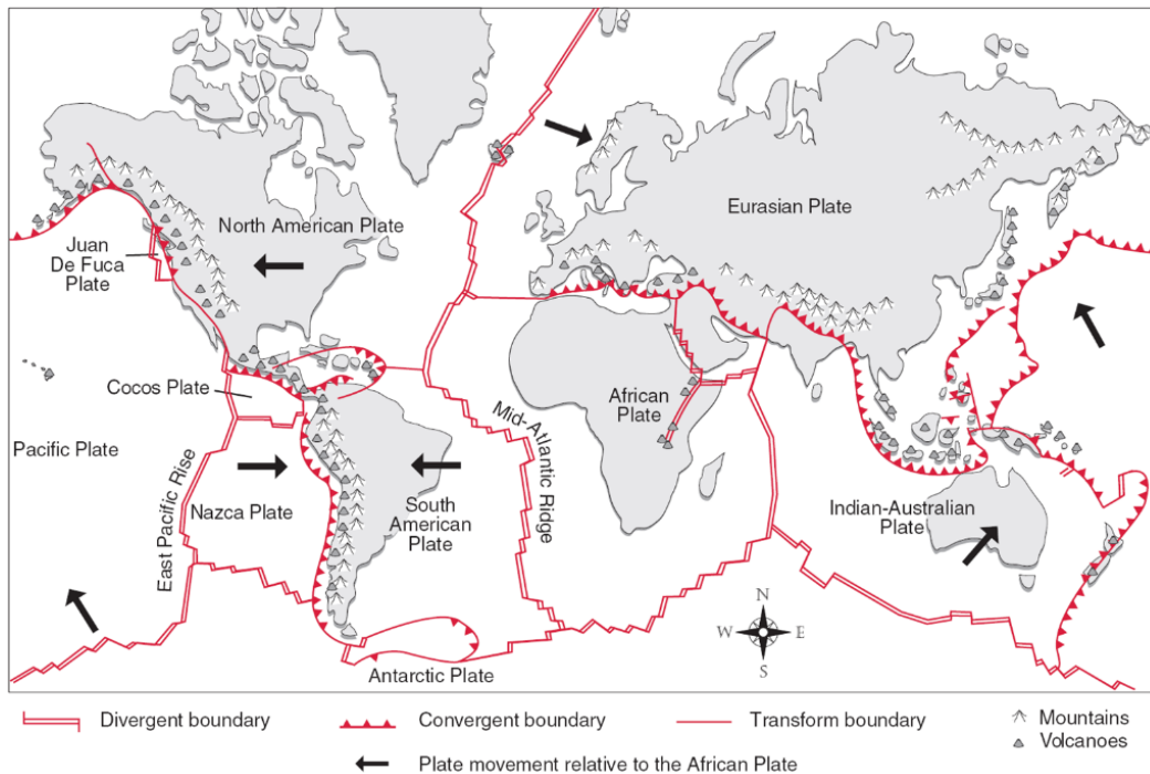
Figura 4.1 Mapa mundi, com a divisão da crosta segundo suas placas siálicas (continentais) e basálticas (oceânicas).
