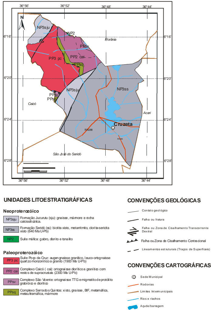
Figura 3 - Mapa Geológico
