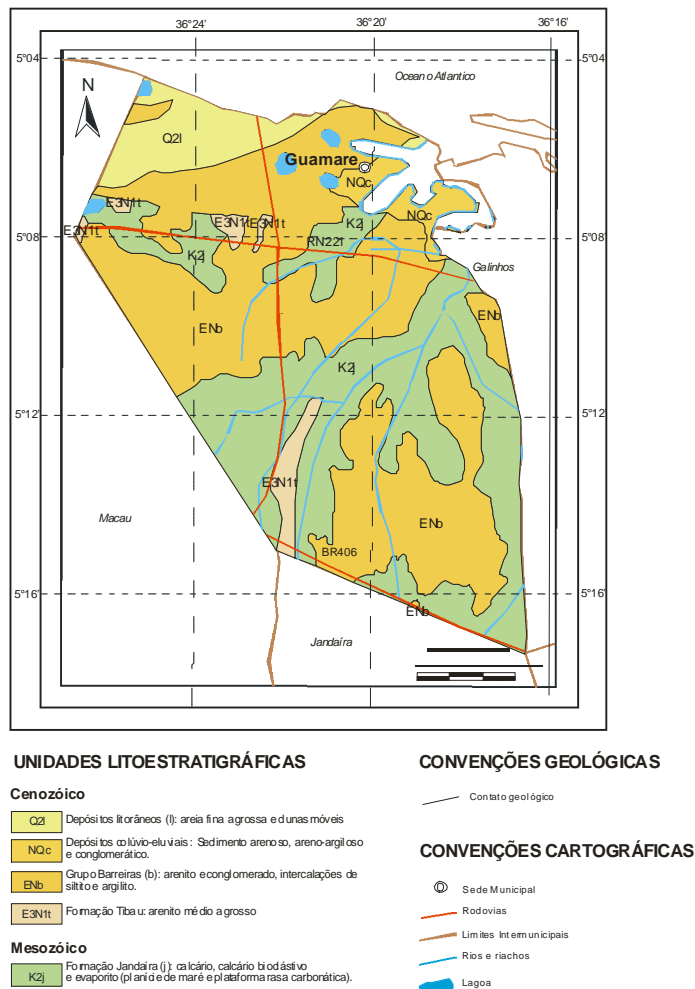
Figura 3 - Mapa Geológico
