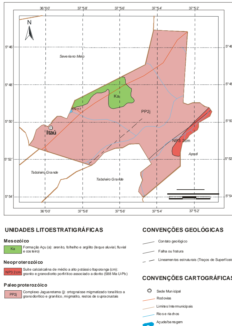
Figura 3 - Mapa Geológico
