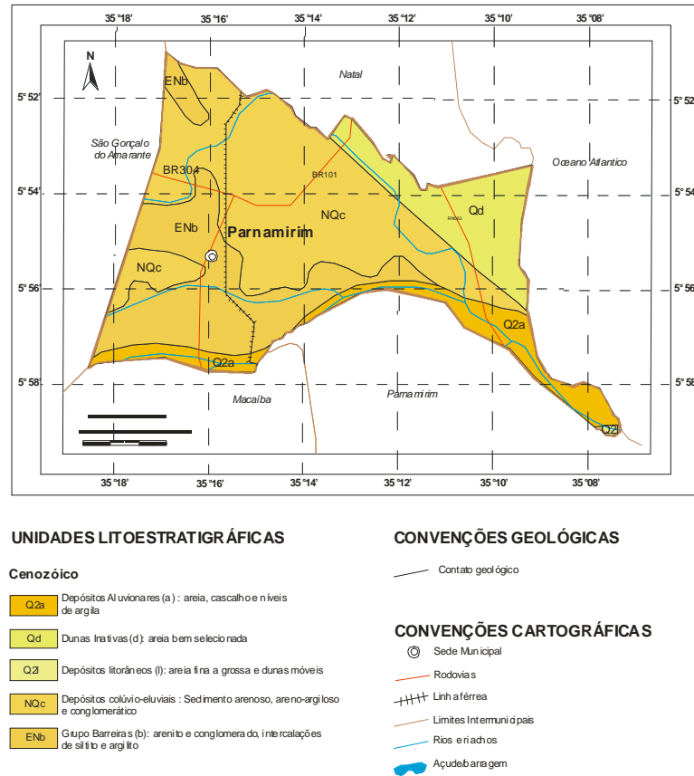
Figura 3 - Mapa Geológico
