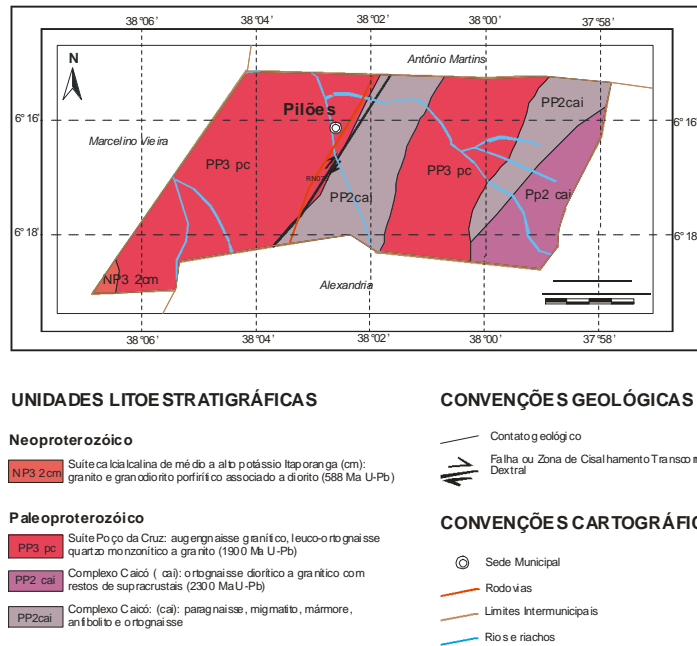
Figura 3 - Mapa Geológico
