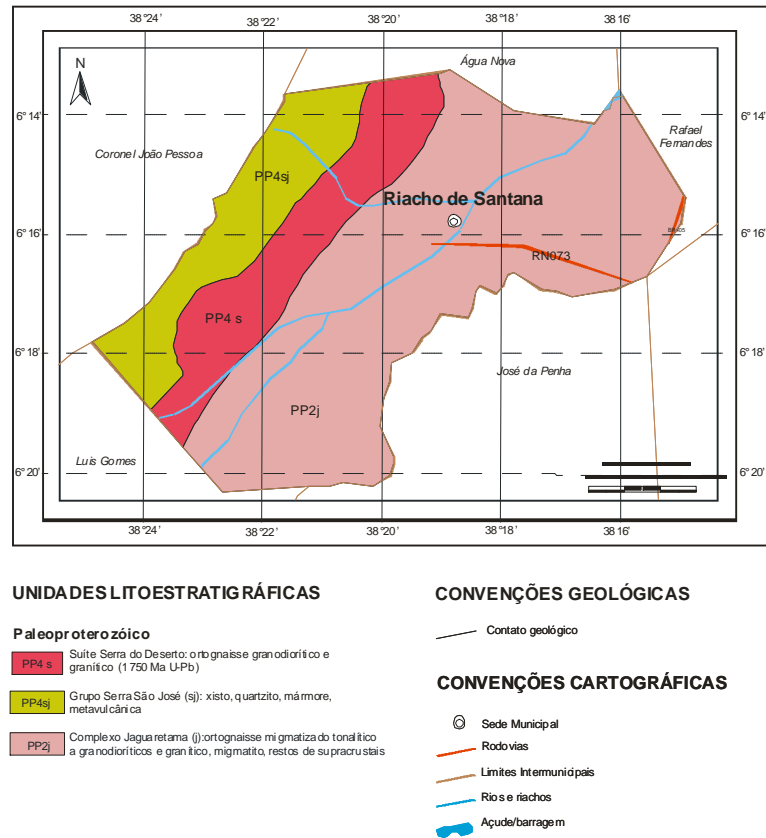
Figura 3 - Mapa Geológico
