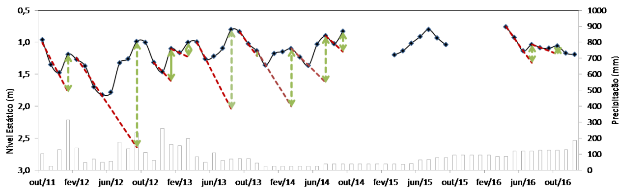
Figura 5 - Nível Estático e Curvas de Recessão Antecedente do Poço Xangrilá (Código SIAGAS: 4300020529). Período: 01/10/2011 a 08/12/2016.
