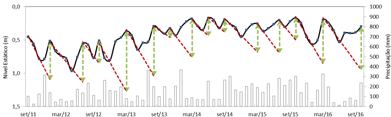
Figura 2 - Nível Estático e Curvas de Recessão Antecedente do Poço Curumim (Código SIAGAS: 4300020526). Período: 09/09/2011 a 15/10/2016.
