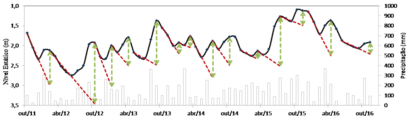
Figura 4 - Nível Estático e Curvas de Recessão Antecedente do Poço Capão da Canoa (Código SIAGAS: 4300020528). Coordenadas: 29°45'17"Sul e 50°02'50"Oeste - Profundidade: 72m - Período: 01/10/2011 a 10/12/2016
