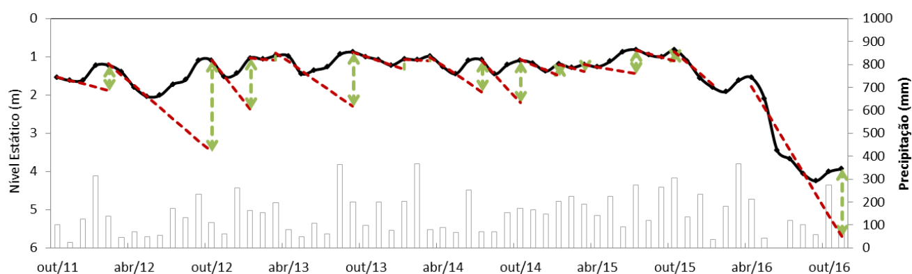
Figura 3 - Nível Estático e Curvas de Recessão Antecedente do Poço São Jorge (Código SIAGAS: 4300020527). Período: 01/10/2011 a 08/12/2016.
