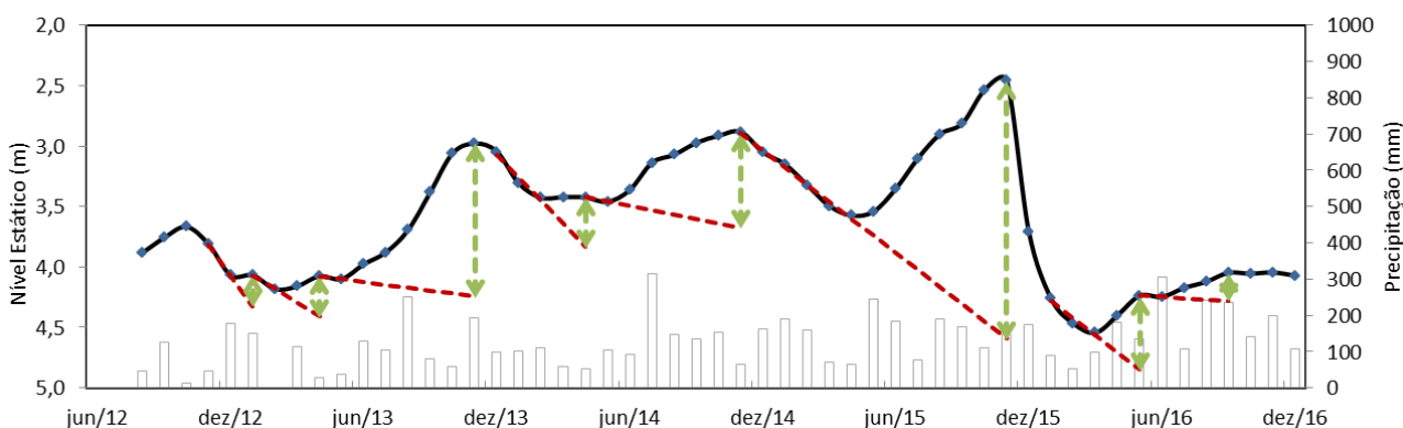
Figura 6 - Nível Estático e Curvas de Recessão Antecedente do Poço Osório (Código SIAGAS: 4300020530). Período: 15/09/2011 a 08/12/2016.
