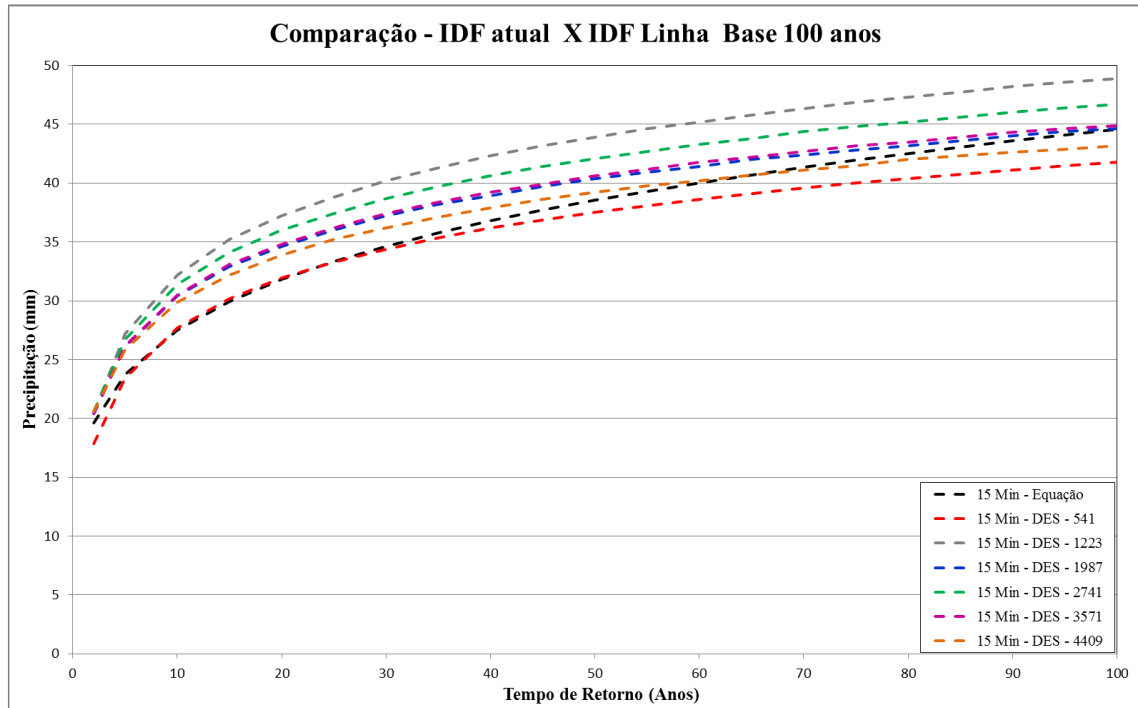
Figura 10. Quantis da IDF atual em preto e quantis IDF Desagregadas para duração de 15 minutos e as seis opções de sementes do LARS-WG.
