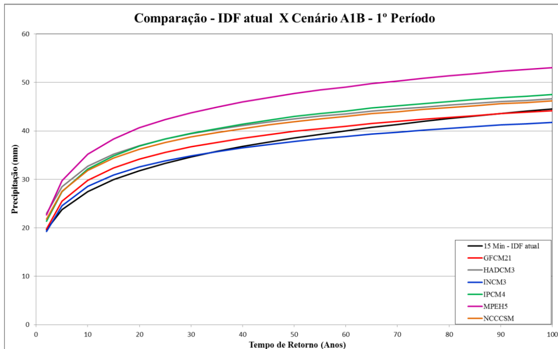
Figura 19. Quantis da IDF atual em preto e quantis IDF Desagregadas para duração de 15 minutos, Cenário A1B, 1º Período, nos seis Modelos Climáticos do LARS-WG.
