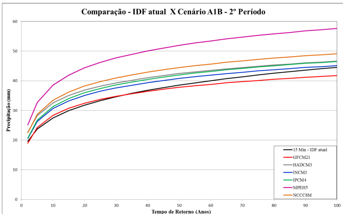
Figura 34. Quantis da IDF atual em preto e quantis IDF Desagregadas para duração de 15 minutos, Cenário A1B, 2º Período, nos seis Modelos Climáticos do LARS-WG.
