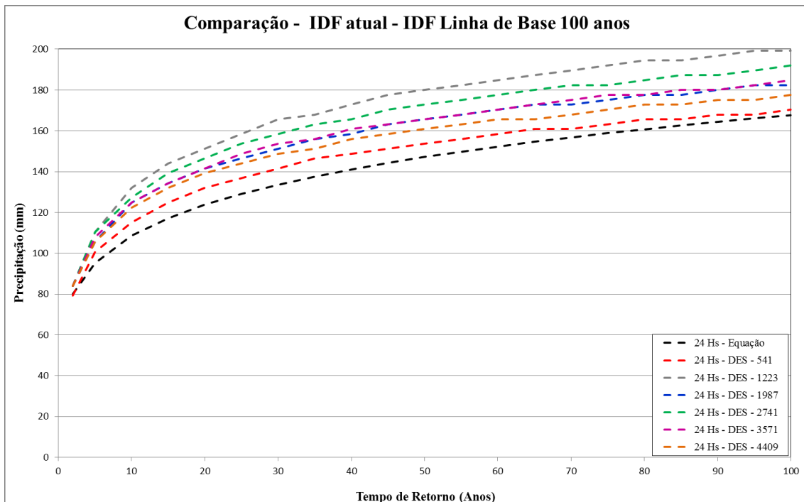
Figura 15. Quantis da IDF atual em preto e quantis IDF Desagregadas para duração de 24 horas e as seis opções de sementes do LARS-WG.
