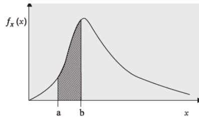
Figura 4. Função Distribuição de Probabilidade (FDP). Fonte: Naghettini e Pinto, 2007.
