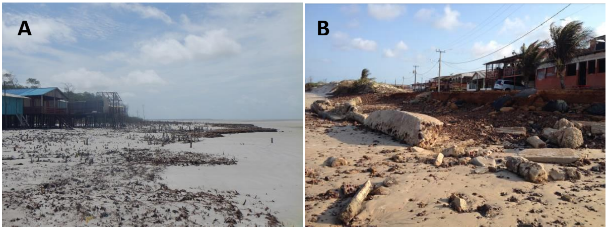
Figura 28: (A) Manguezal soterrado por deposição de sedimentos arenosos na praia do Crispim, em 2016. (B) Destruição de rua beira-mar a partir do recuo da linha de costa na praia do Crispim, no ano de 2015.
