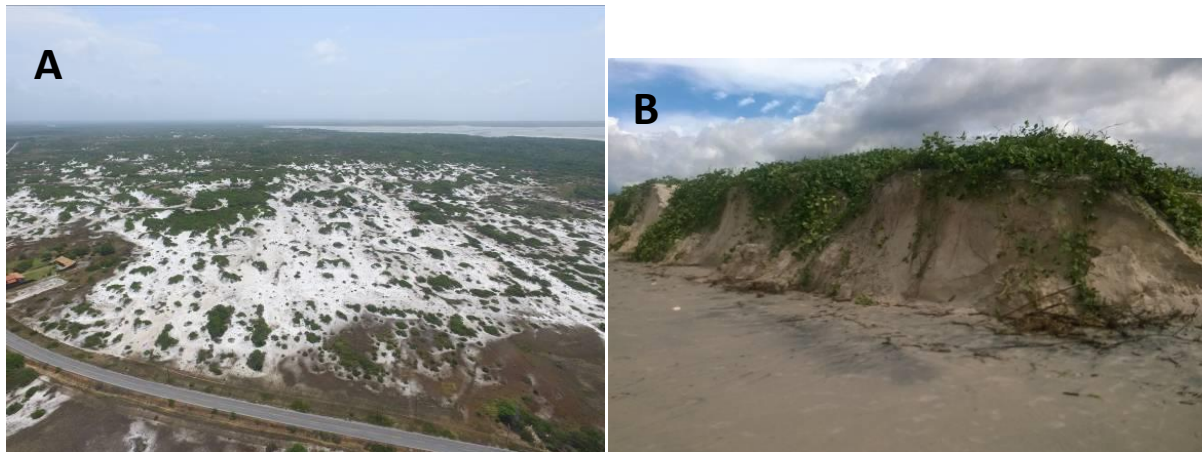
Figura 21- (A) Paleodunas recortada por estrada de acesso à praia do Crispim. (B) Dunas frontais verticalizadas existentes na região central da praia do Crispim em 2015.
