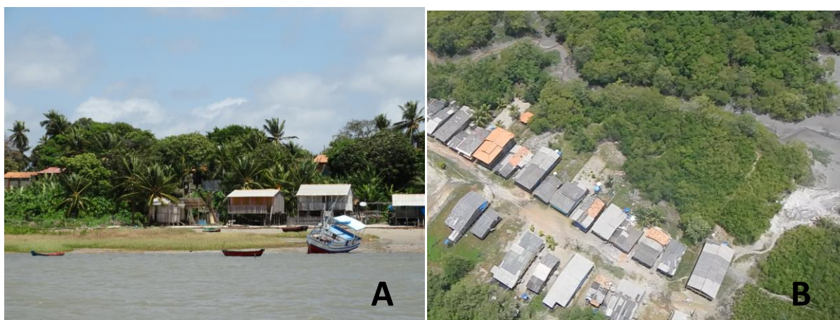
Figura 46- (A) Moradias instaladas em planície fluviomarina, (B) Imagem aérea da área de manguezal na vila de Marudá em 2017.
