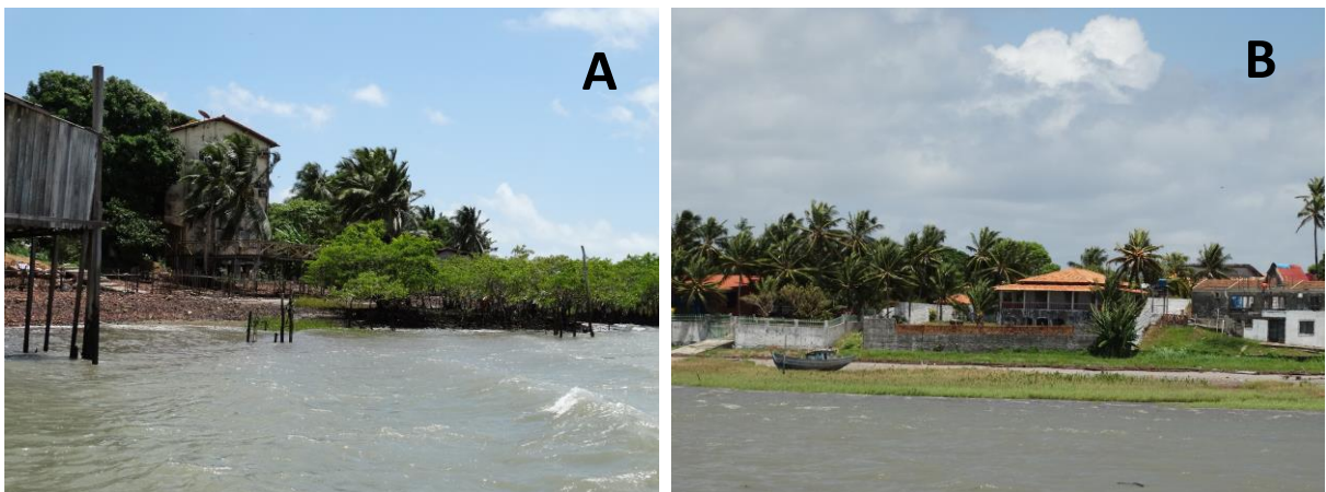
Figura 54- (A) Região com ausência de obras de contenção diariamente inundada protegida da ação erosiva pela vegetação de mangue. (B) Setor sem obra de contenção e vegetação totalmente exposto aos agentes costeiros, na orla marítima de Marudá, em 2017.
