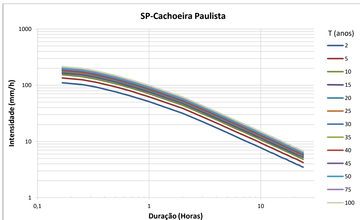
Figura 02 – Curvas intensidade-duração-frequência
