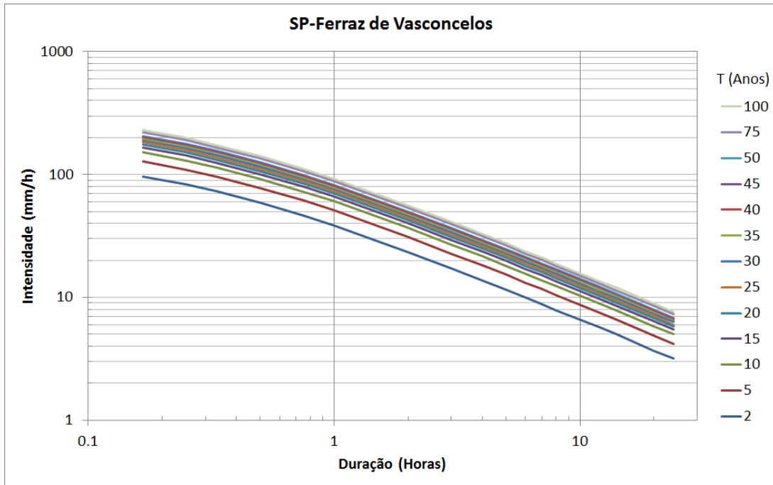
Figura 02 – Curvas intensidade-duração-freqüência
