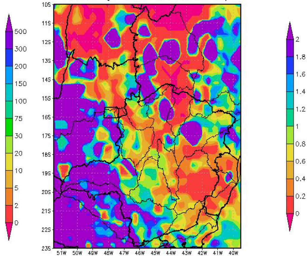
Figura 3 - Razão entre o total precipitado de agosto de 2016 a média histórica de 1998 a 2014.
