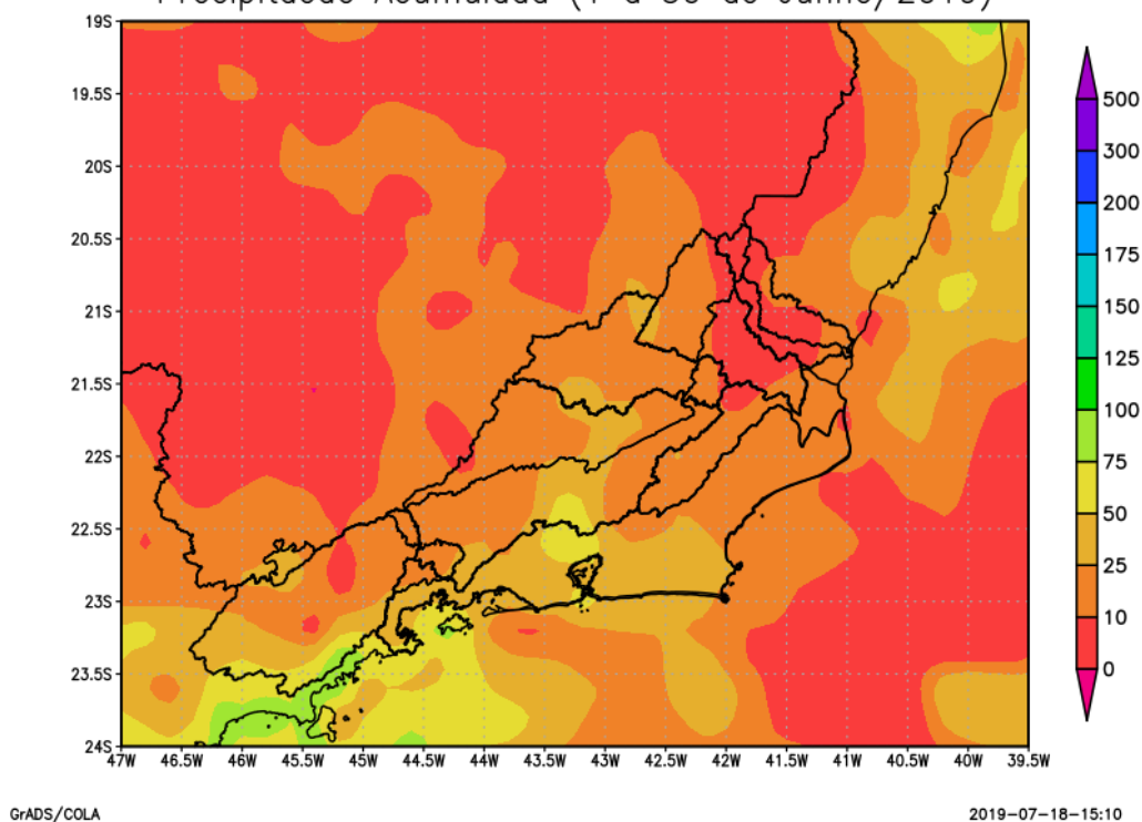
Figura 2 - Precipitação acumulada no mês de junho de 2019.
