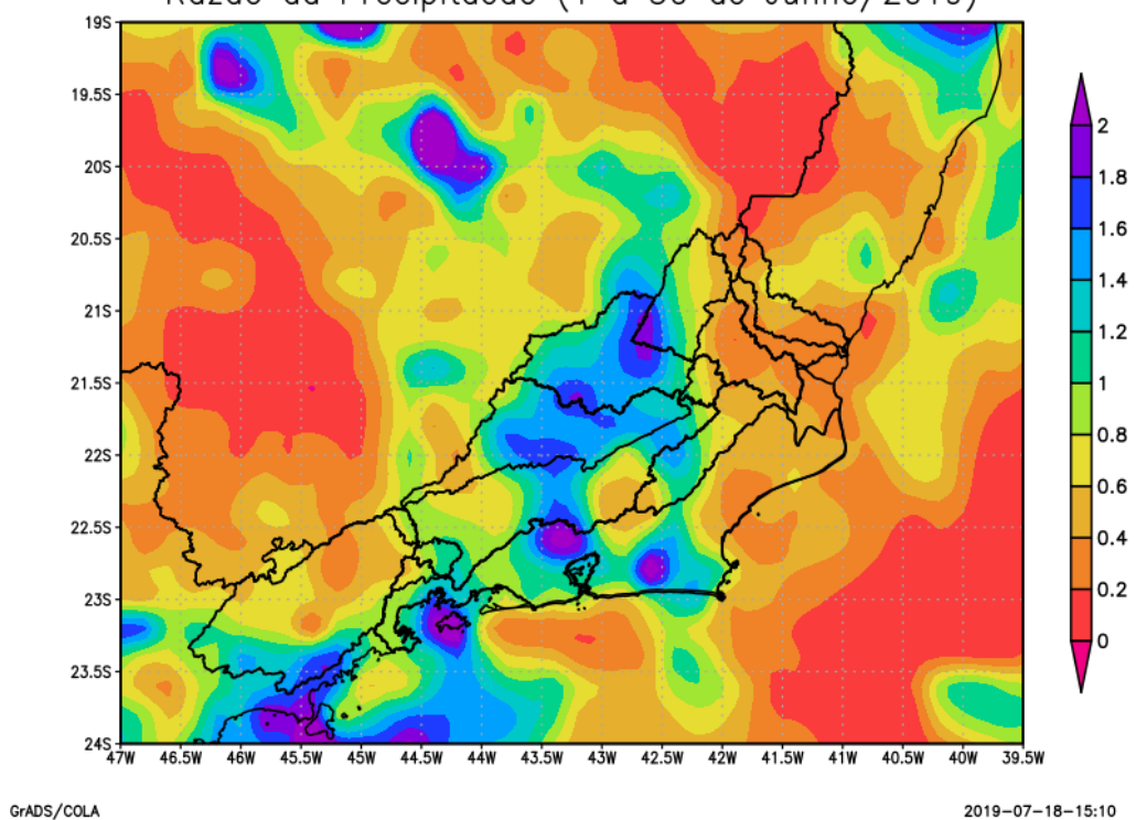
Figura 3 – Razão entre a precipitação acumulada no mês de junho de 2019 e a média histórica de junho (1998 a 2013).
