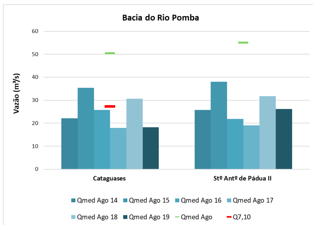
Figura 8 – Comparação entre a vazão média de agosto de 2014, 2015, 2016, 2017, 2018 e 2019, média histórica de agosto e vazão de referência Q_{7,10} nas estações da Bacia do Rio Pomba
