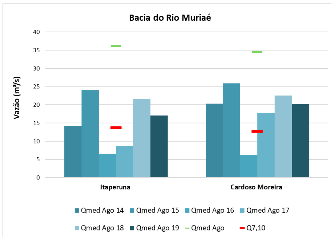
Figura 7 – Comparação entre a vazão média de agosto de 2014, 2015, 2016, 2017, 2018 e 2019, média histórica de agosto e vazão de referência Q_{7,10} nas estações da Bacia do Rio Muriaé
