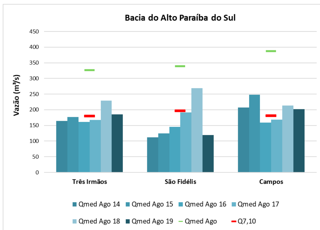
Figura 9 – Comparação entre a vazão média de agosto de 2014, 2015, 2016, 2017, 2018 e 2019, média histórica de agosto e vazão de referência Q 7,10 nas estações da Bacia do Alto Paraíba do Sul
