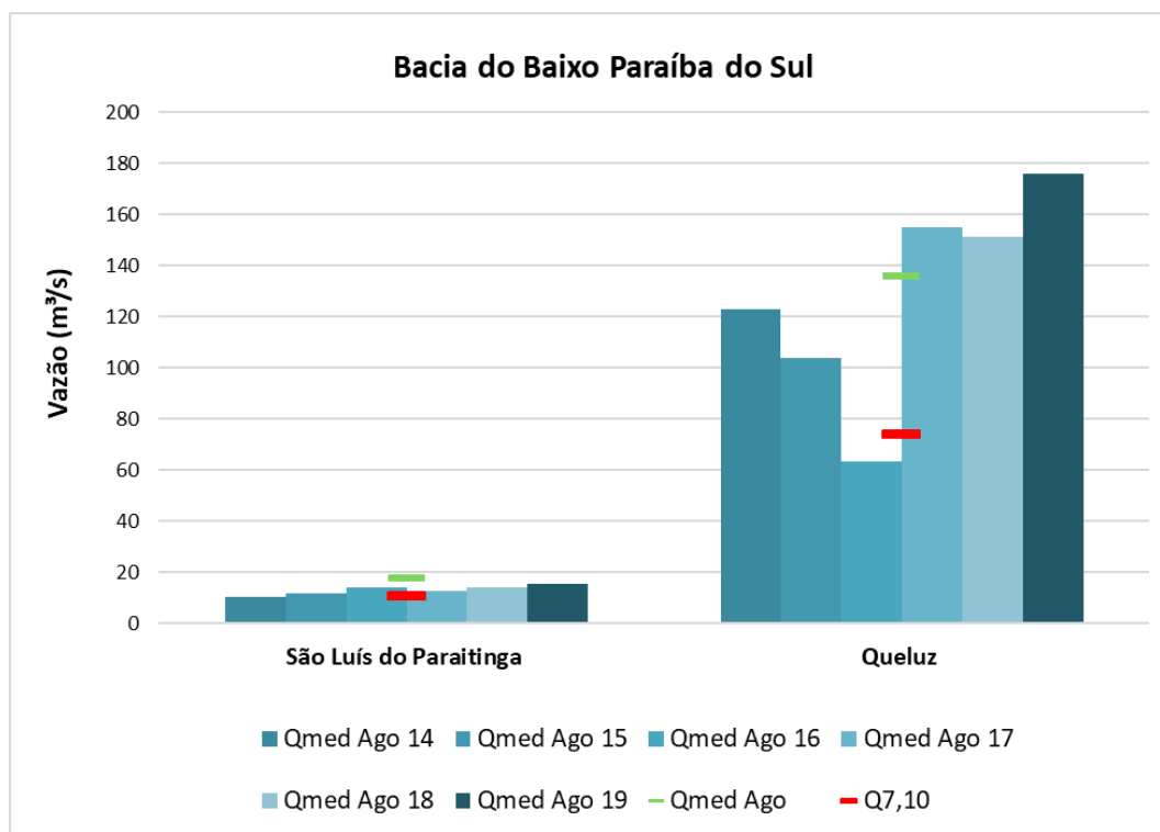
Figura 11 – Comparação entre a vazão média de agosto de 2014, 2015, 2016, 2017, 2018 e 2019, média histórica de agosto e vazão de referência Q_{7,10} nas estações da Bacia do Baixo Paraíba do Sul
