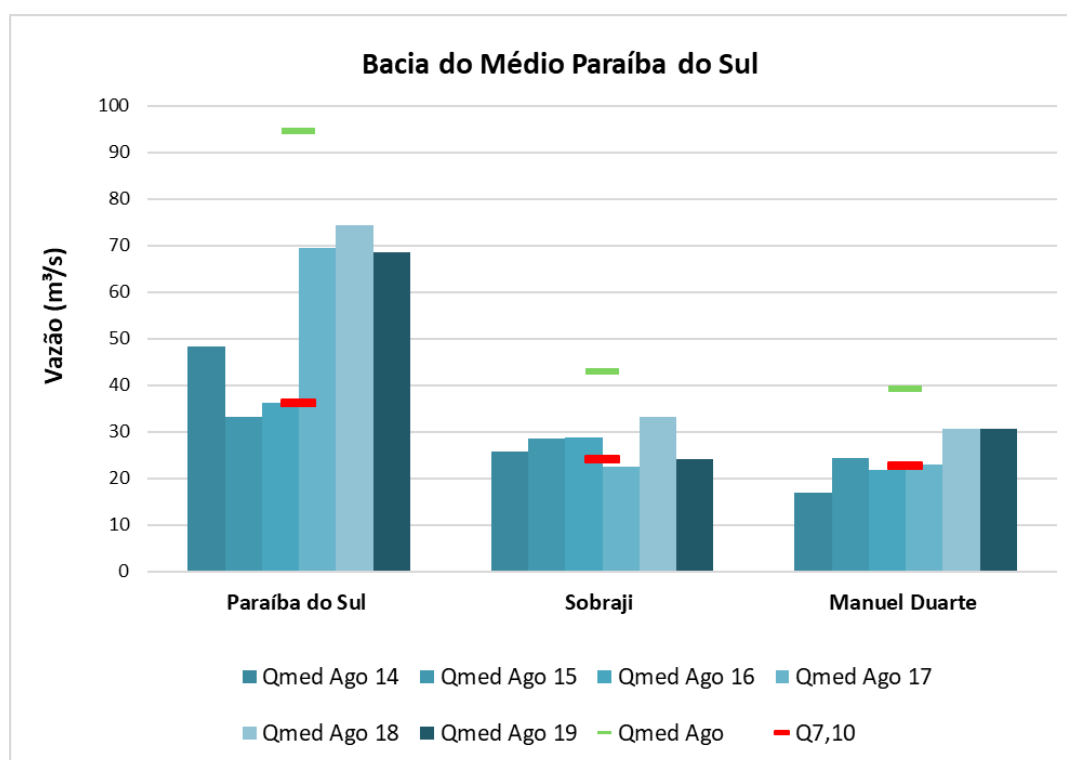
Figura 10 – Comparação entre a vazão média de agosto de 2014, 2015, 2016, 2017, 2018 e 2019, média histórica de agosto e vazão de referência Q 7,10 nas estações da Bacia do Médio Paraíba do Sul
