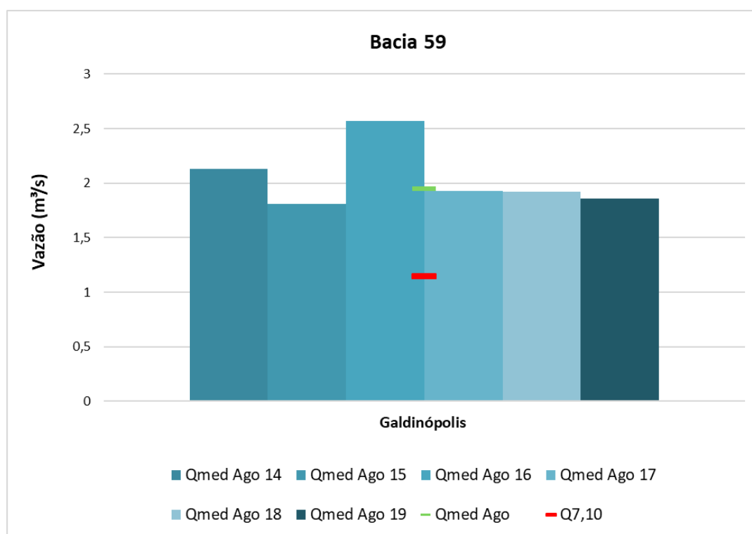
Figura 12 – Comparação entre a vazão média de agosto de 2014, 2015, 2016, 2017, 2018 e 2019, média histórica de agosto e vazão de referência Q_{7,10} nas estações da Bacia 59
