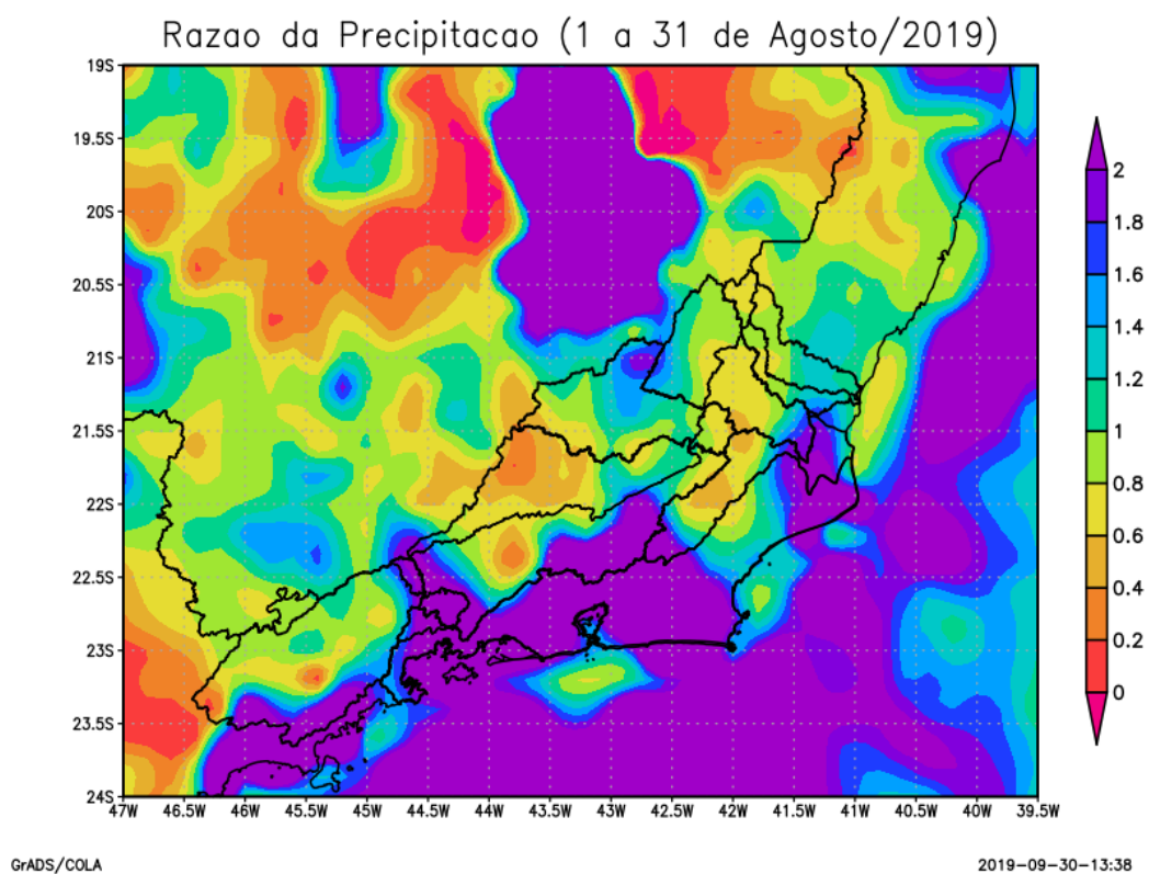
Figura 3 – Razão entre a precipitação acumulada no mês de agosto de 2019 e a média histórica de agosto (1998 a 2013).
