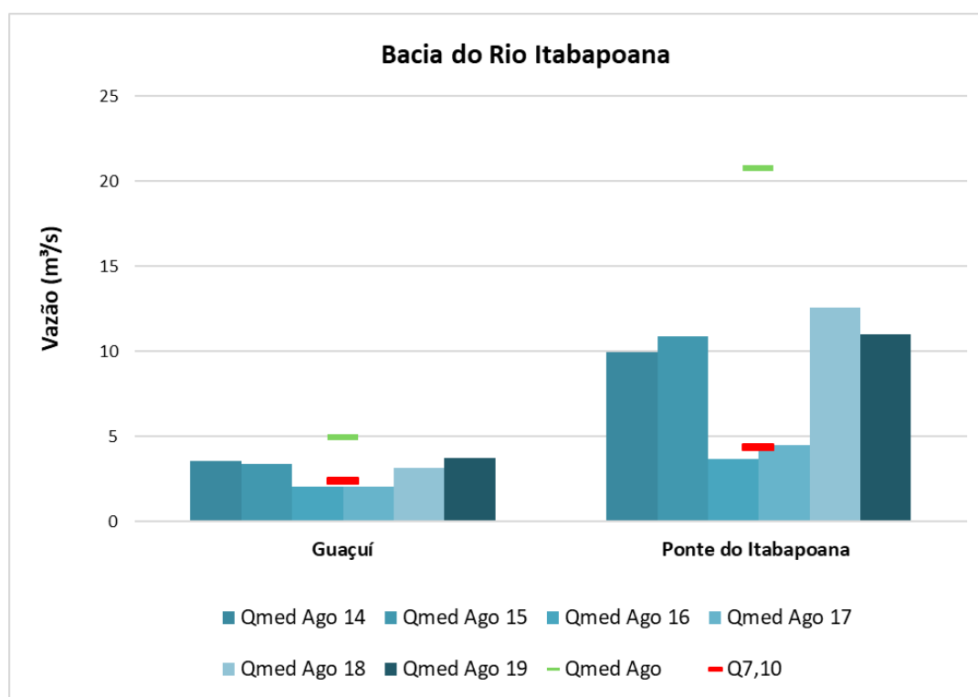
Figura 6 – Comparação entre a vazão média de agosto de 2014, 2015, 2016, 2017, 2018 e 2019, média histórica de agosto e vazão de referência Q_{7,10} nas estações da Bacia do Rio Itabapoana
