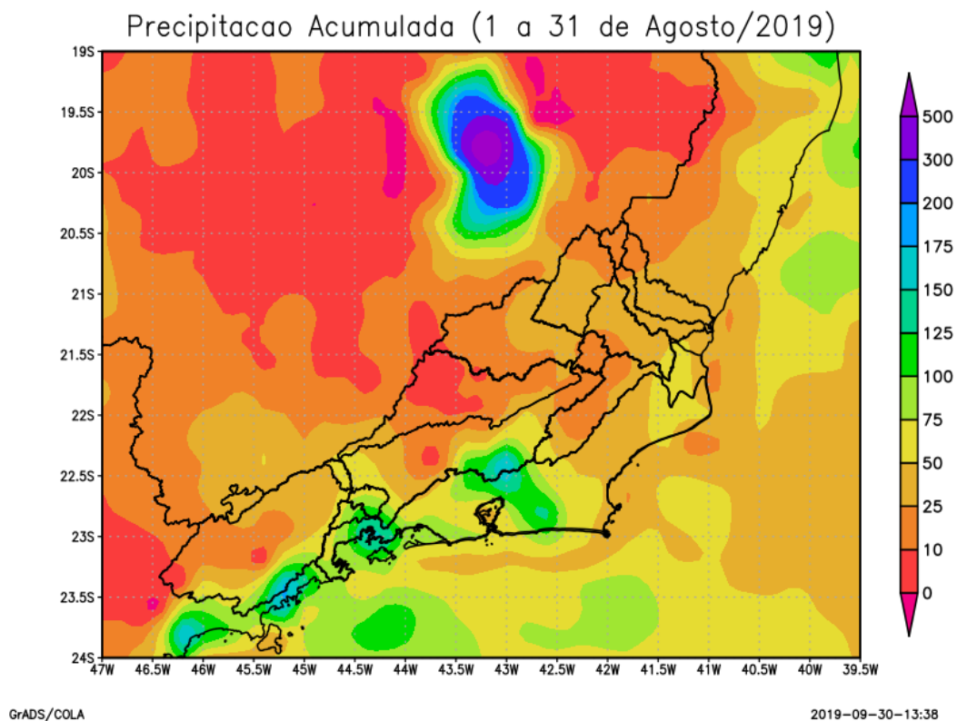
Figura 2 - Precipitação acumulada no mês de agosto de 2019.
