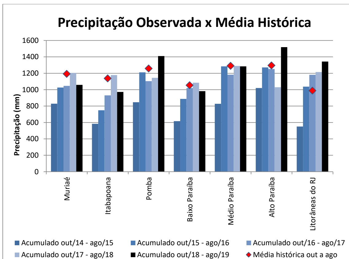
Figura 4 - Comparação entre a precipitação média histórica de outubro a agosto, a precipitação acumulada de outubro de 2014 a agosto de 2015, outubro de 2015 a agosto de 2016, outubro de 2016 a agosto de 2017, outubro de 2017 a agosto de 2018, e outubro de 2018 a agosto de 2019 nas bacias da área de atuação da SUREG/SP.
