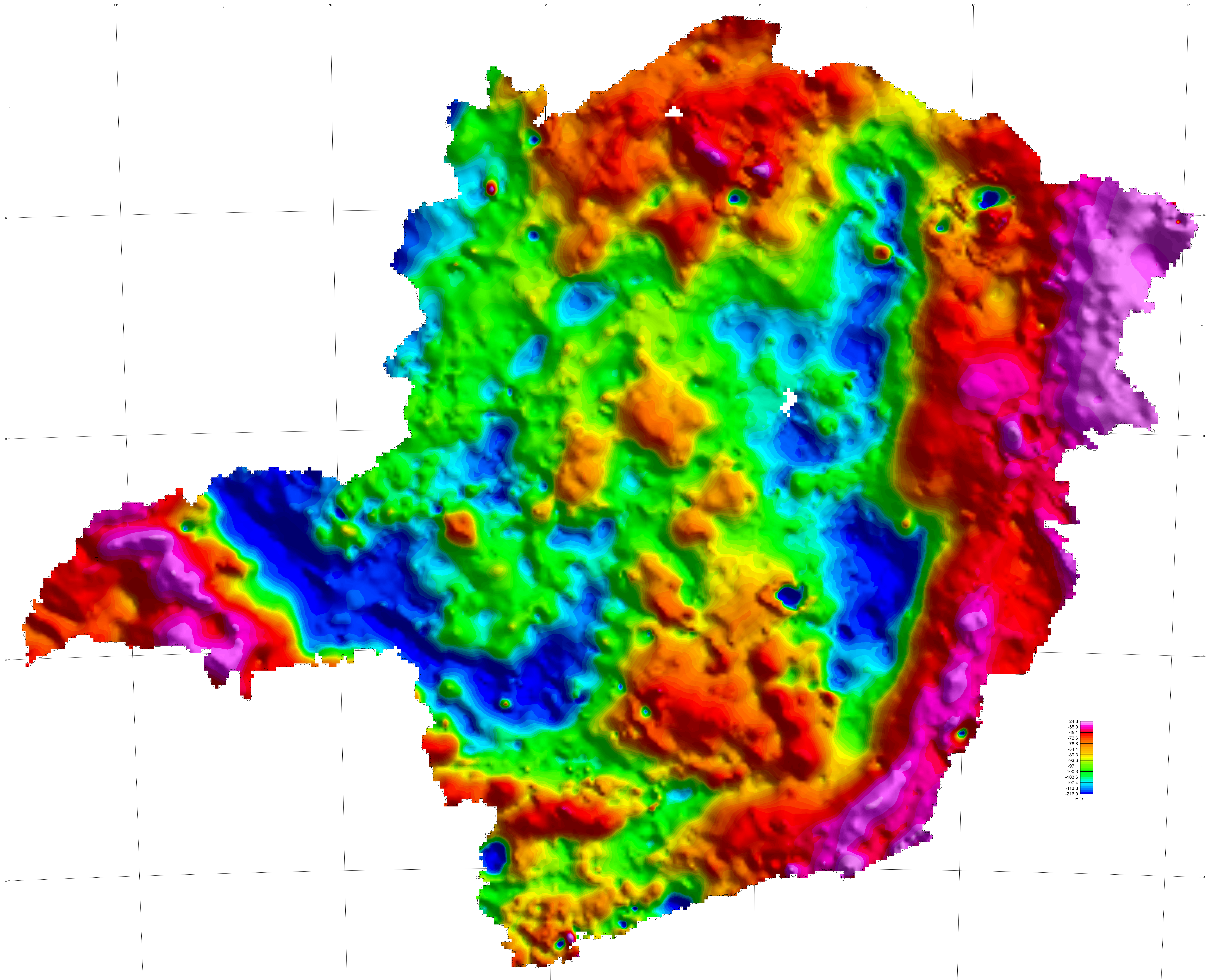
ATLAS AEROGEOFÍSICO DO ESTADO DE MINAS GERAIS - ANOMALIA BOUGUER ESCALA 1:1.000.000 PROJEÇÃO POLICÔNICA Equador - Meridiano Central: 50° W, G. Datum Horizontal: SIRGAS 2000
