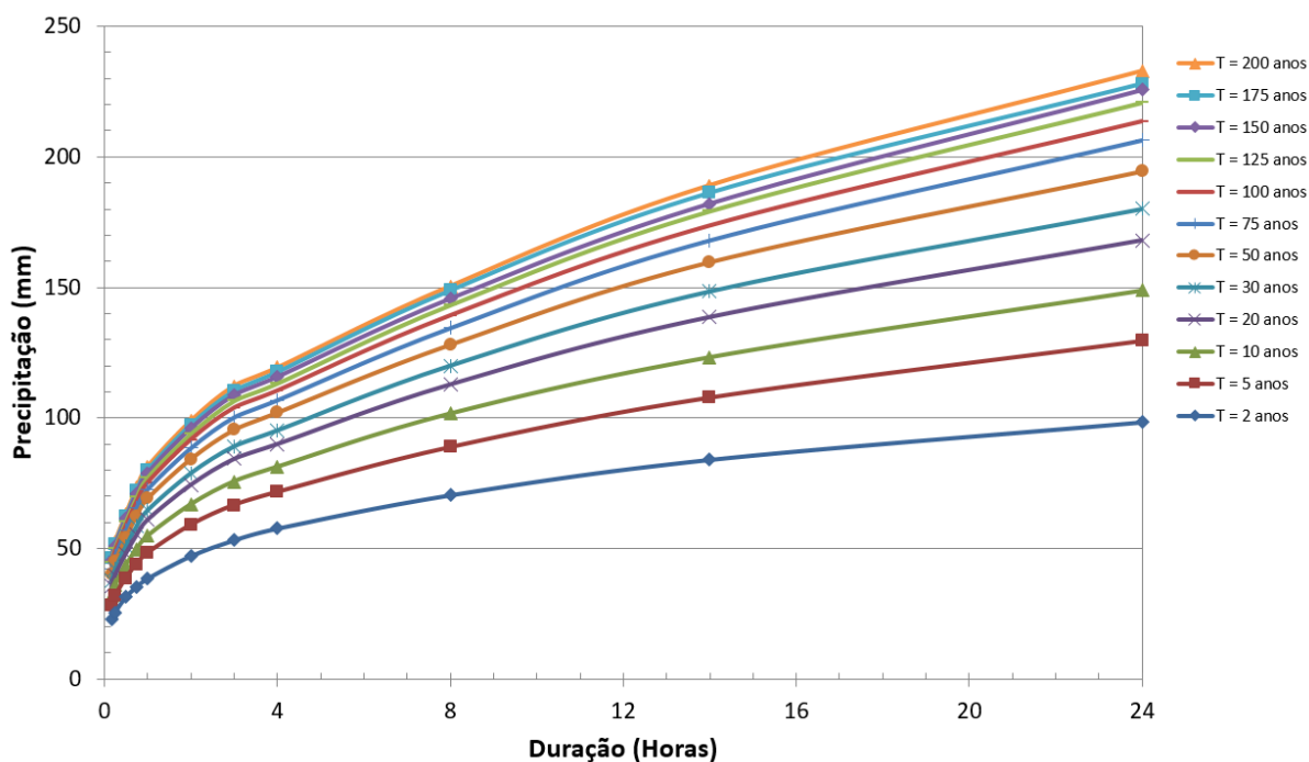
Figura 04 – Curvas Altura-Duração-Freqüência (PA de 1450mm).
