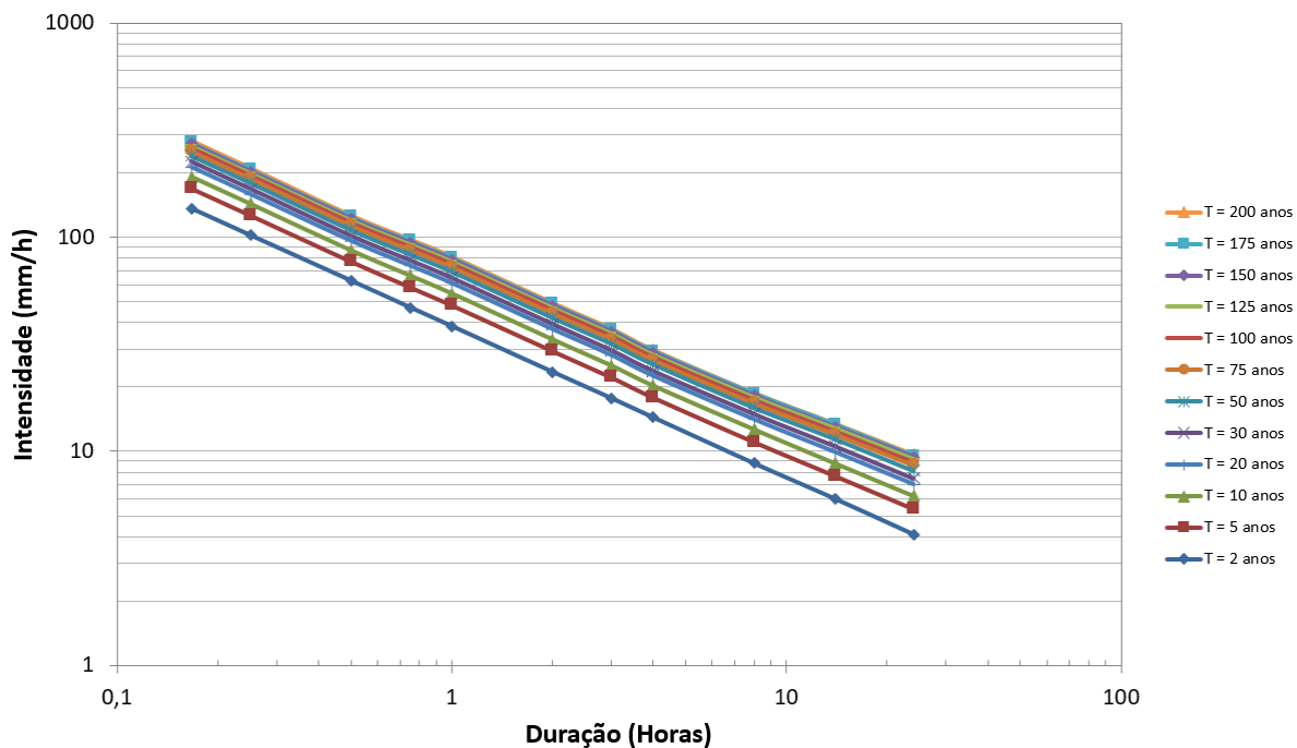
Figura 03 – Curvas Intensidade-Duração-Freqüência (PA de 1450mm).
