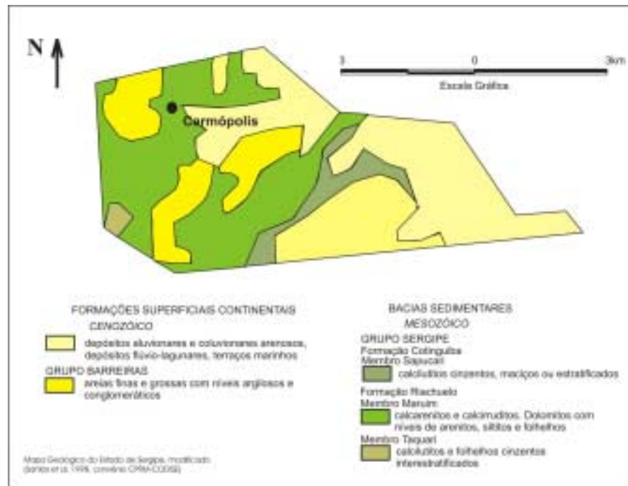
Figura 2 – Geologia simplificada do município
