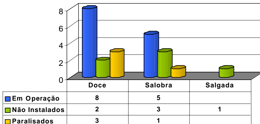
Figura 14 – Qualidade das águas subterrâneas nos aquíferos tipo granular
