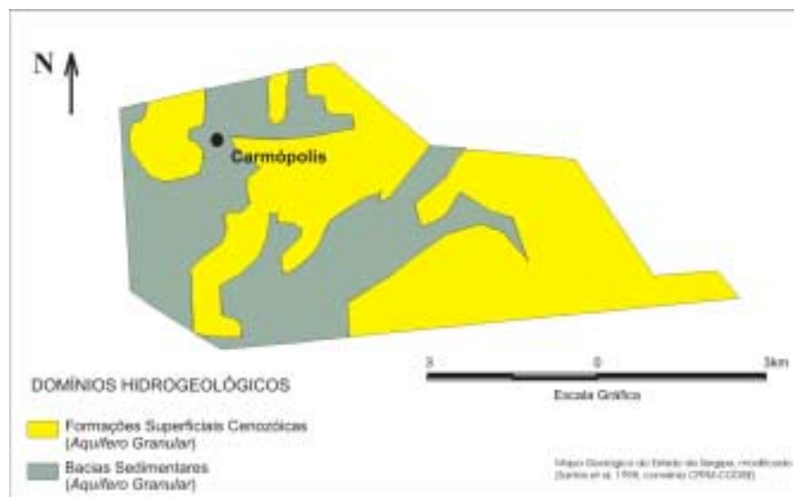
Figura 3 – Domínios hidrogeológicos do município
