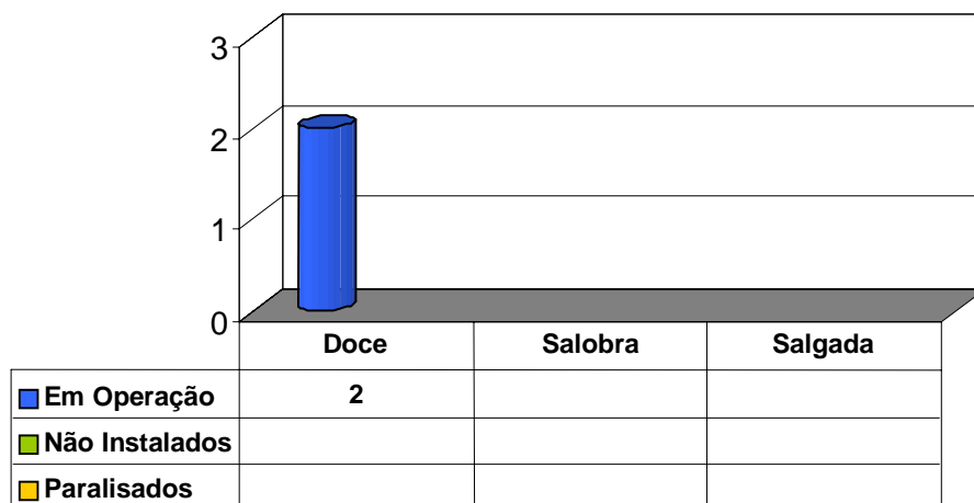
Figura 13 – Qualidade das águas subterrâneas nos aquíferos tipo fissural
