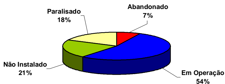
Figura 7 – Situação dos poços cadastrados
