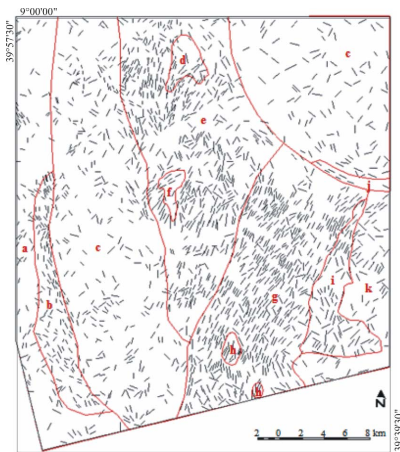
Figura 6-7 – Mapa de zonas homólogas de relevo. 9°20'55\"
