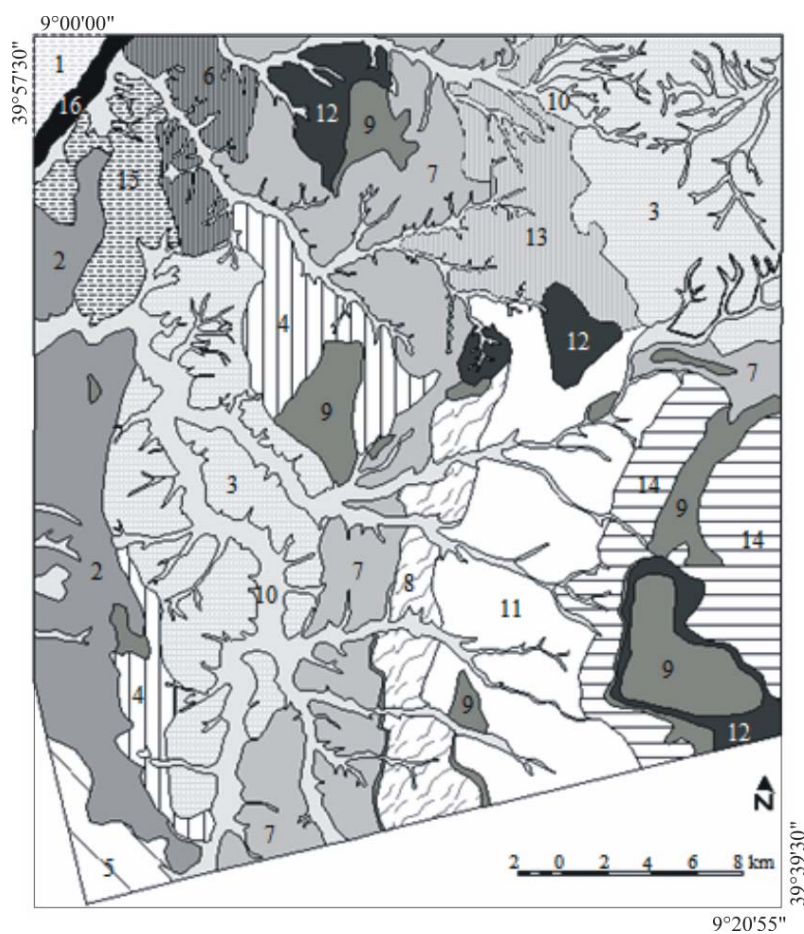
Figura 6-8 – Mapa de zonas homólogas de tonalidade.
