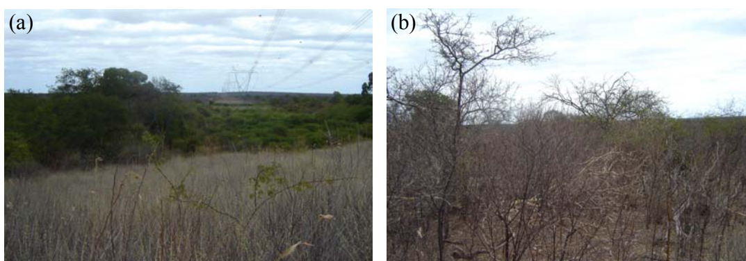
Figura 4-4 – Aspectos da vegetação da área de estudo. (a) Contraste da vegetação verde no aluvião com a vegetação seca do biotita-gnaisse; (b) Vegetação densa e seca do quartzo-mica xisto.
