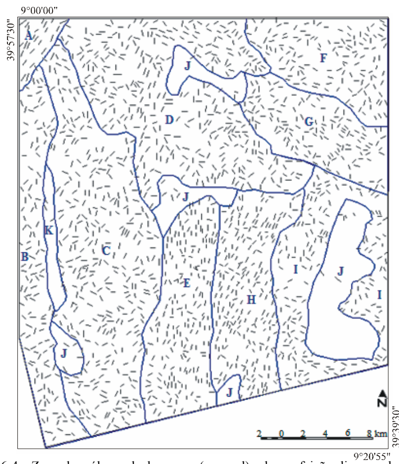
Figura 6-4 – Zonas homogêneas de drenagem (em azul) sobre as feições lineares de drenagem.
