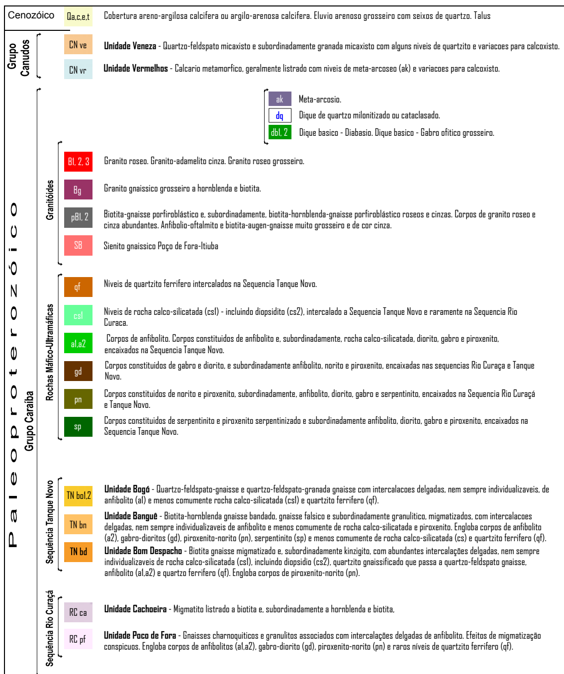
Figura 4-9 – Coluna Litoestratigráfica do mapa geológico do Vale do Rio Curaça (Figura 4.8). Fonte: modificado de Delgado e Souza (1975).
