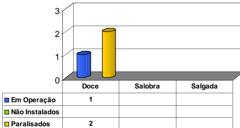
Figura 15 – Qualidade das águas subterrâneas nos aquíferos tipo granular
