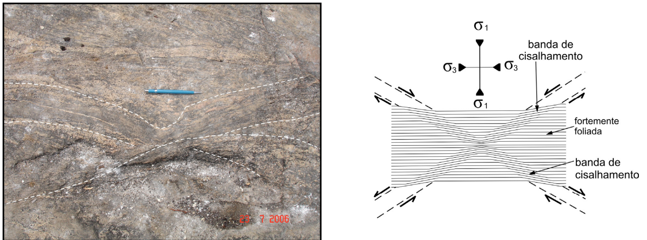
Figura 4.10. Biotita hornblenda granodiorito com banda de cisalhamento conjugada. Afloramento CC-23.
